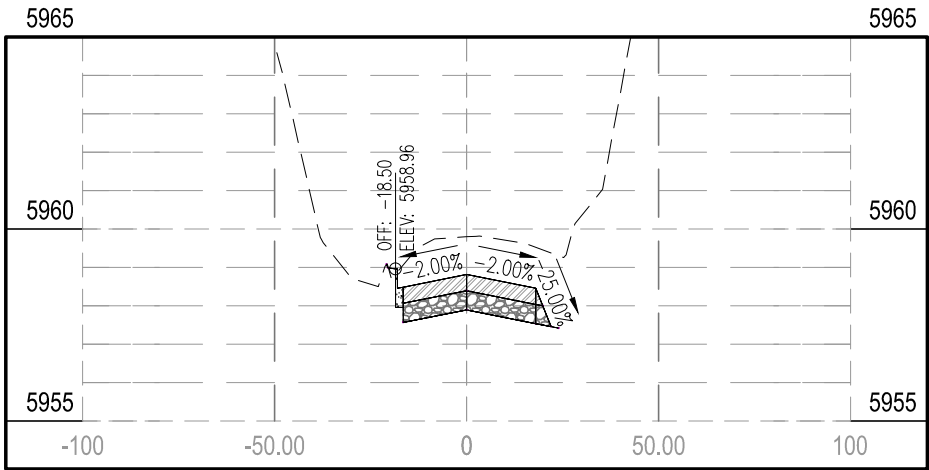
STA 19+75.00
