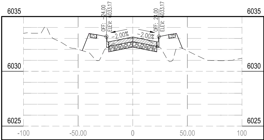
STA 50+00.00
