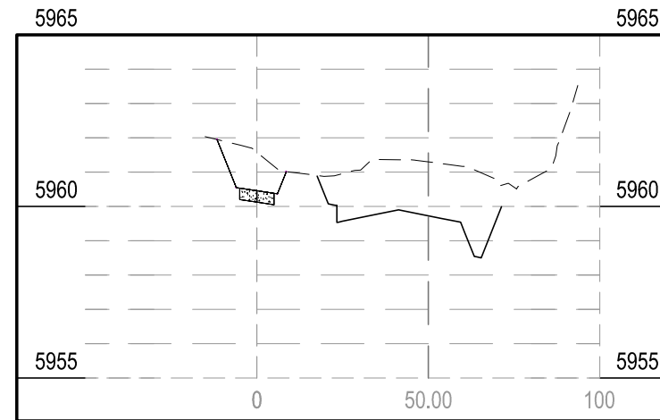
STA 17+00.00
