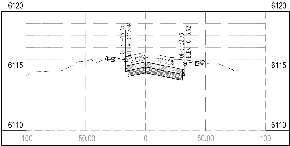
STA 6+00.00
