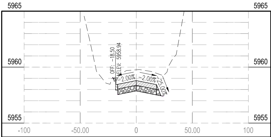
STA 19+78.74
