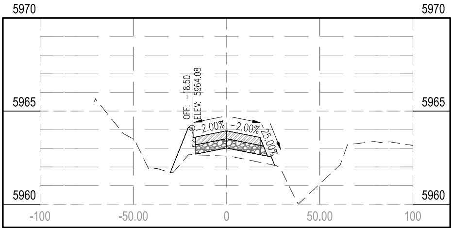
STA 9+50.00
