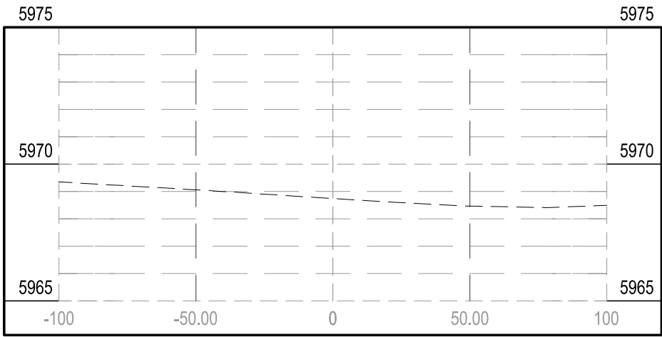
STA 0+50.00
