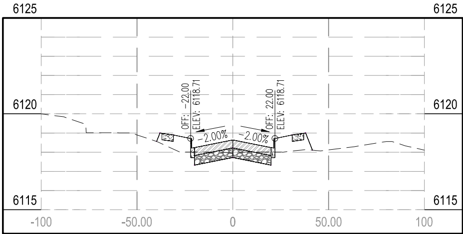
STA 2+00.00
