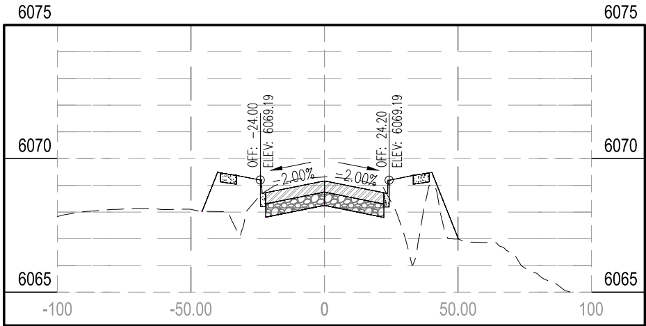
STA 29+00.00
