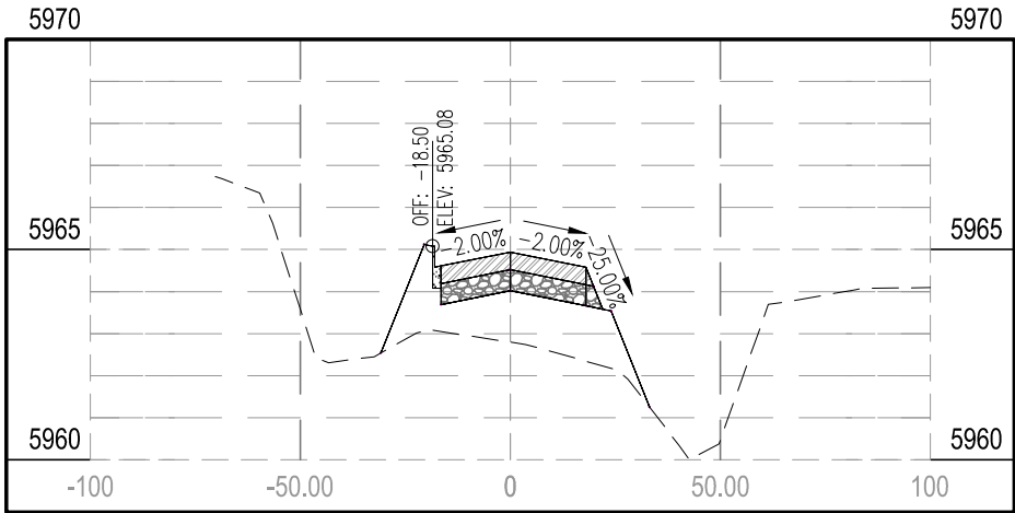
STA 7+50.00
