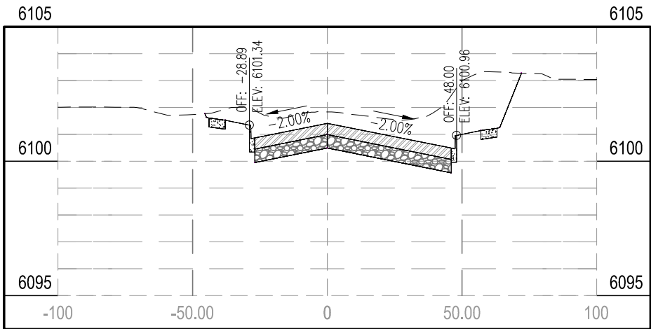
STA 19+00.00
