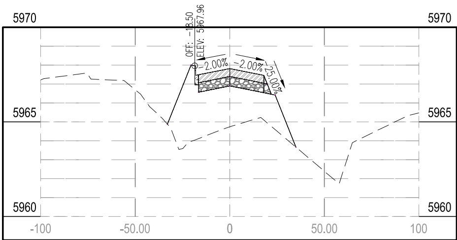
STA 1+75.00
