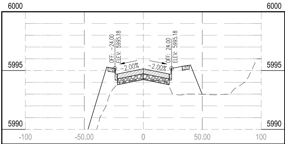
STA 97+00.00
