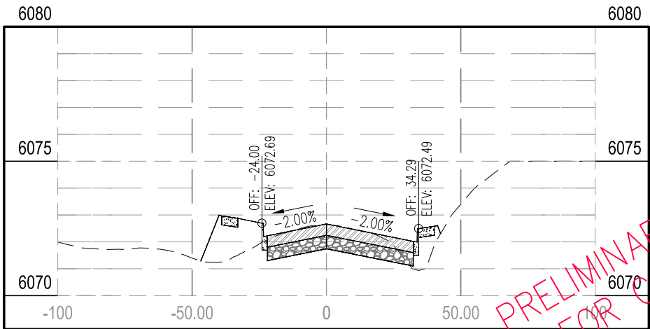
STA 28+00.00
