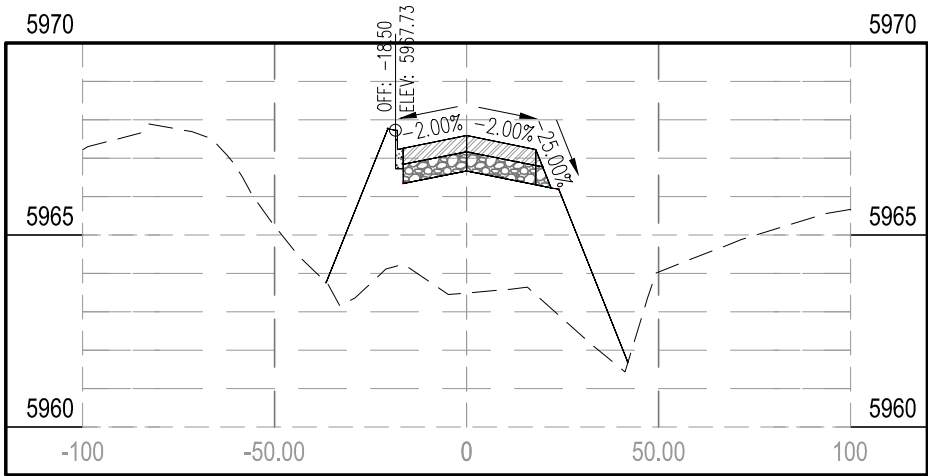
STA 2+20.52
