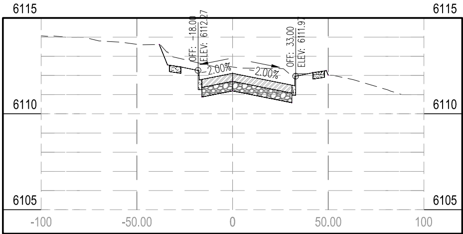
STA 11+00.00
