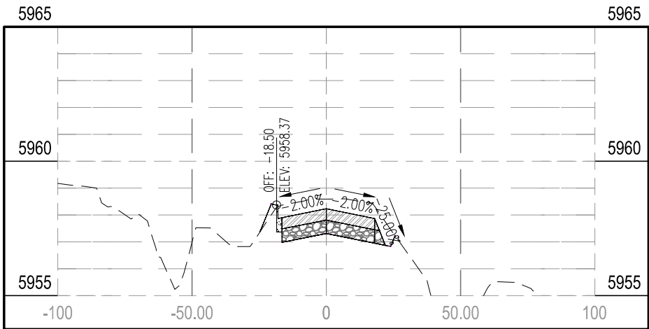
STA 24+32.93
