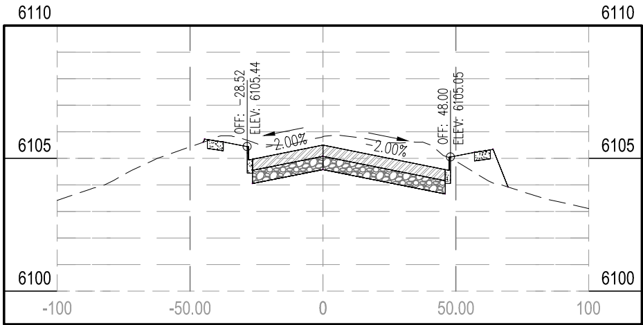
STA 18+00.00
