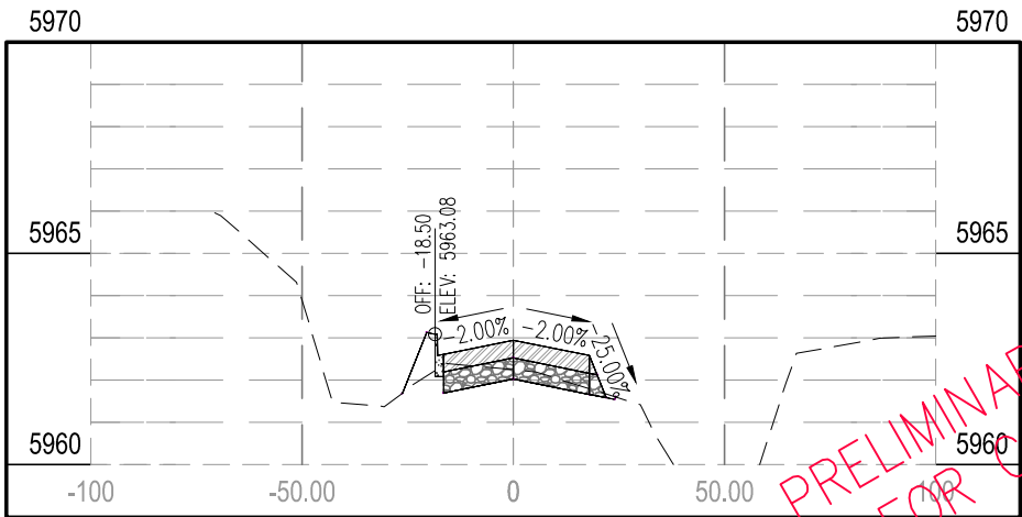
STA 11+50.00
