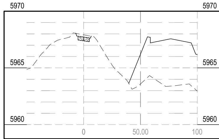
STA 1+52.59
