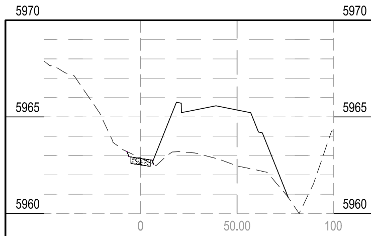
STA 5+55.51
