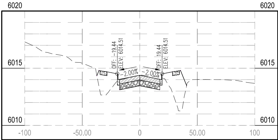
STA 57+00.00
