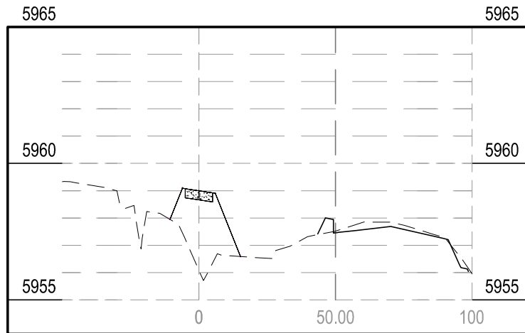
STA 24+00.00
