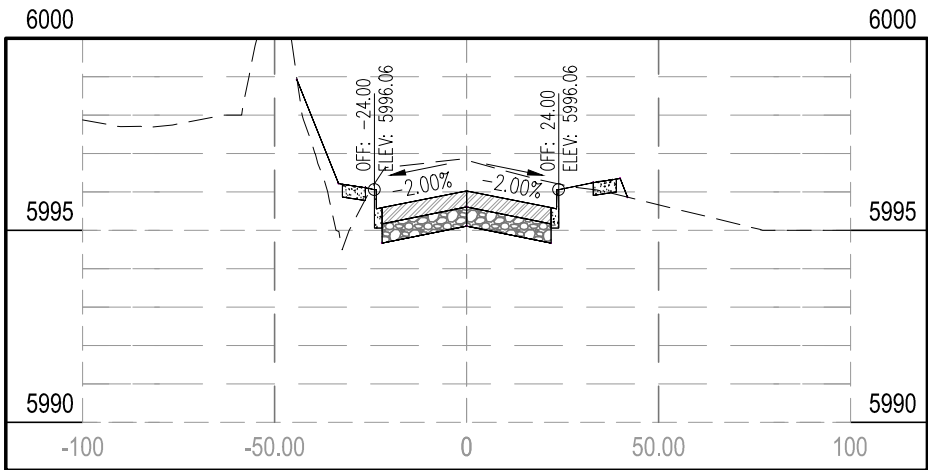
STA 91+00.00
