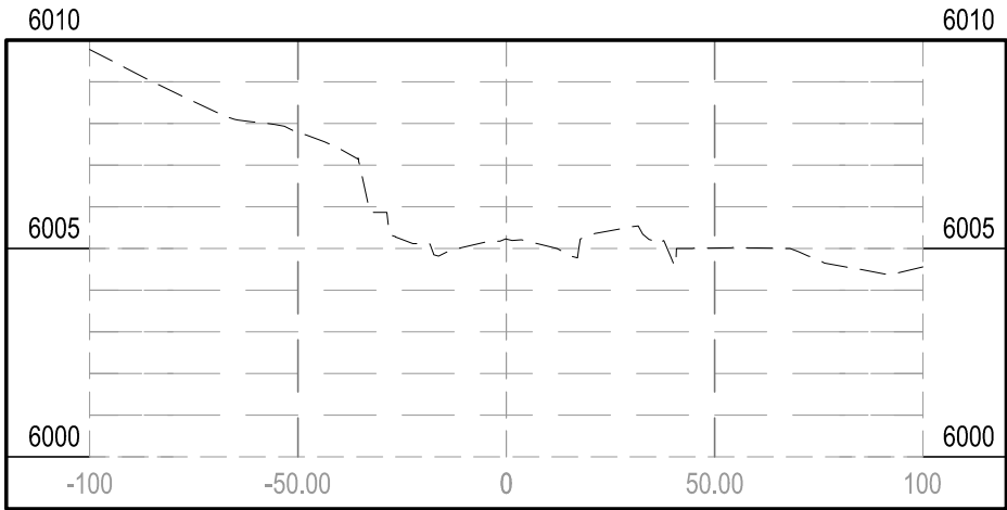
STA 1+00.00
