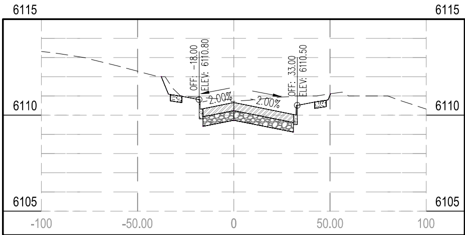
STA 13+00.00
