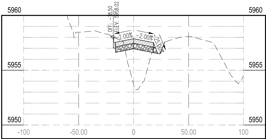
STA 22+00.00
