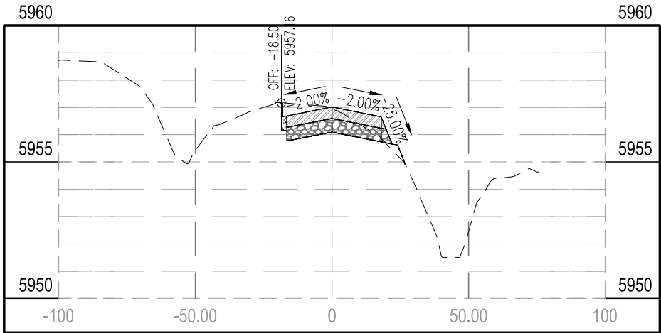
STA 25+50.00
