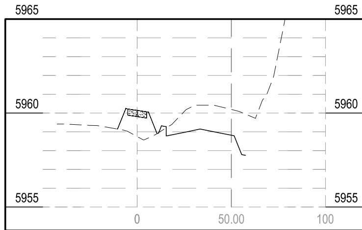
STA 18+50.00
