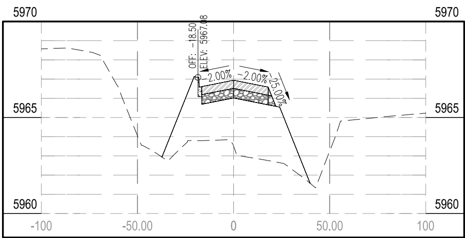
STA 3+50.00
