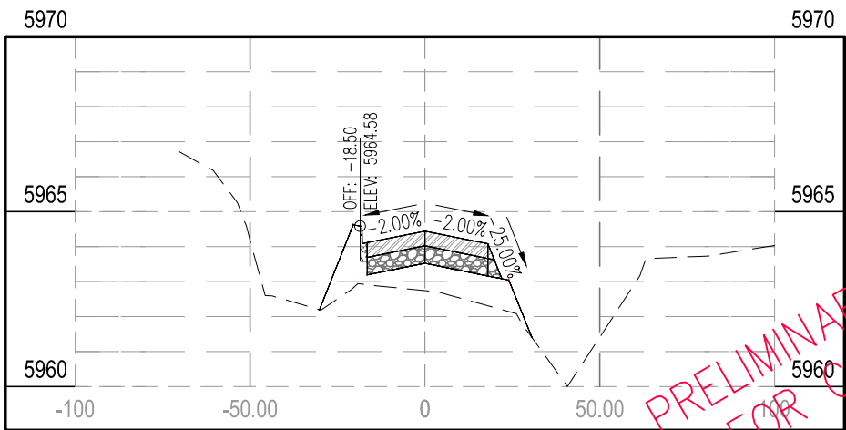
STA 8+50.00
