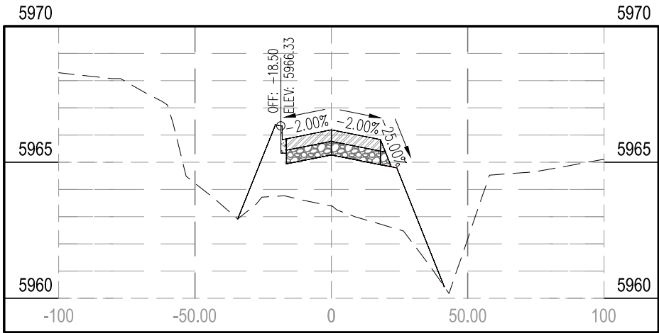
STA 5+00.00
