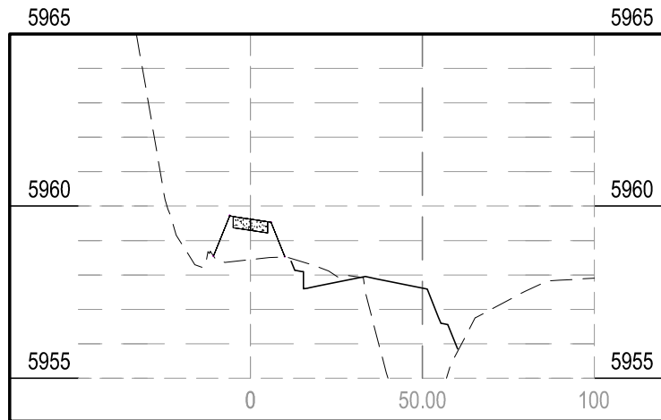
STA 21+00.00
