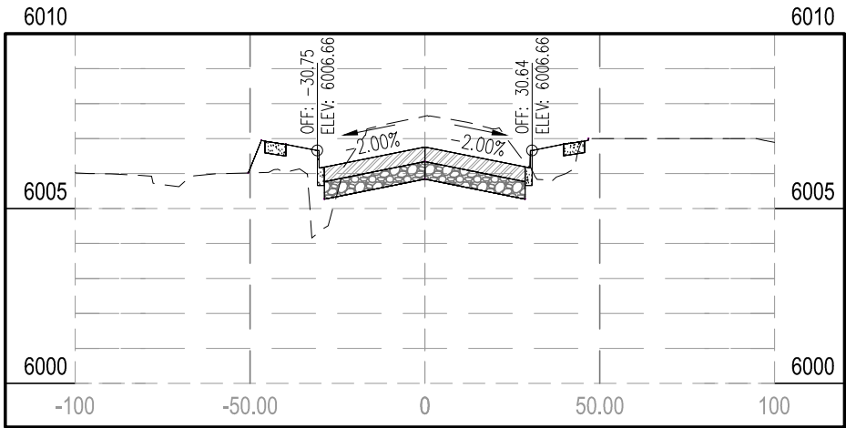
STA 60+00.00
