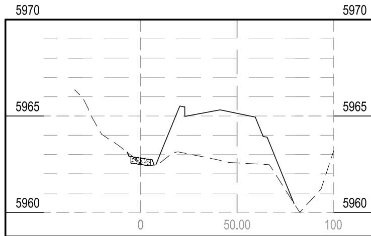
STA 6+00.00
