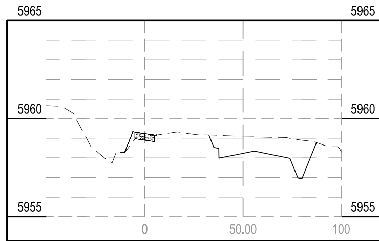
STA 22+86.49
