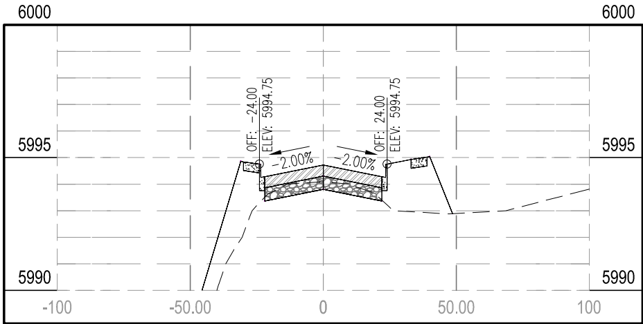
STA 98+00.00
