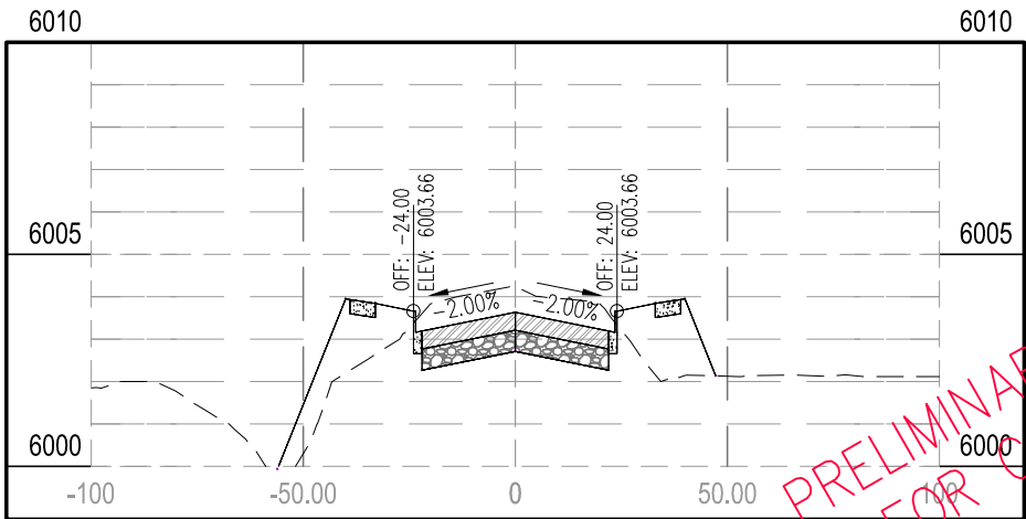
STA 64+00.00
