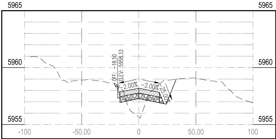
STA 23+00.00
