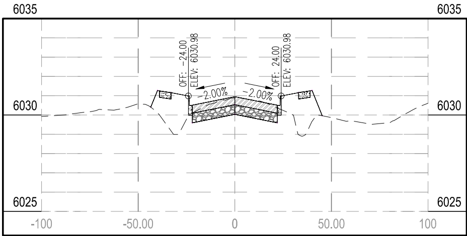
STA 51+00.00
