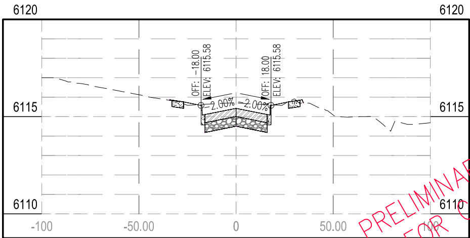
STA 2+50.00
