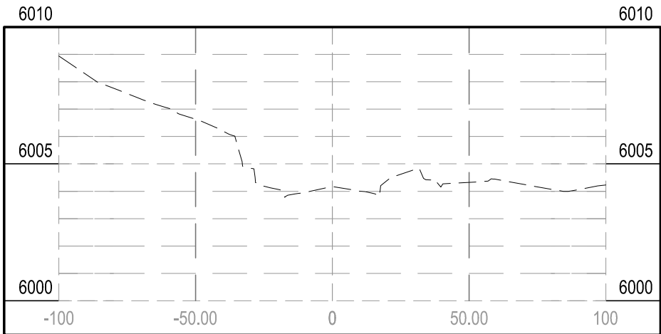
STA 0+50.00
