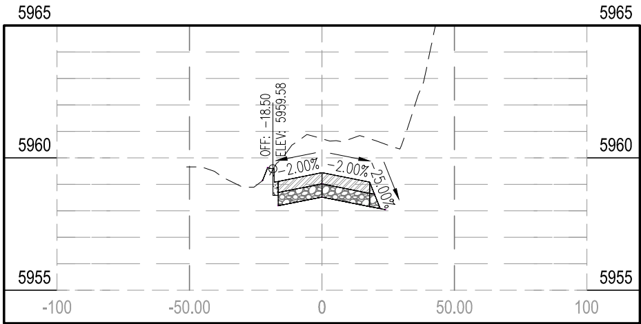
STA 18+50.00
