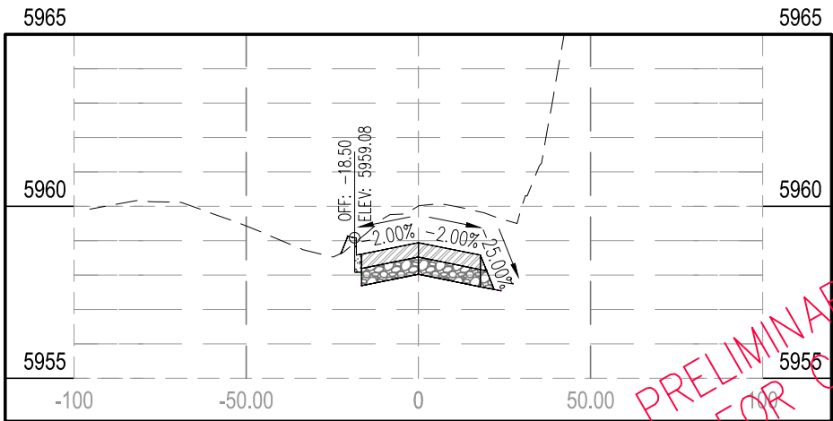
STA 19+50.00
