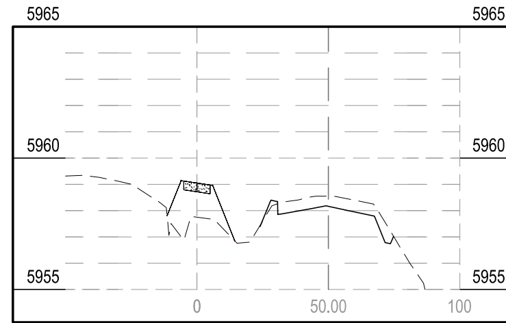
STA 23+75.00
