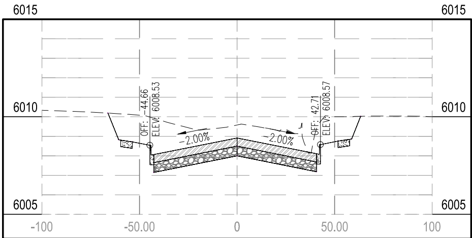
STA 59+00.00
