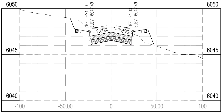
STA 39+00.00
