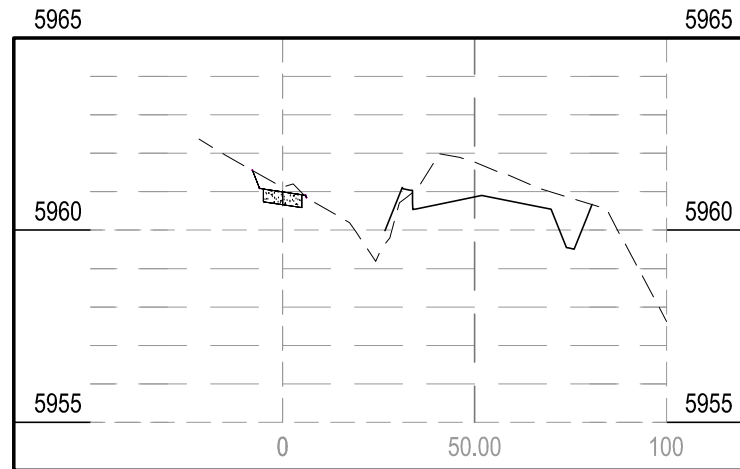
STA 15+00.00
