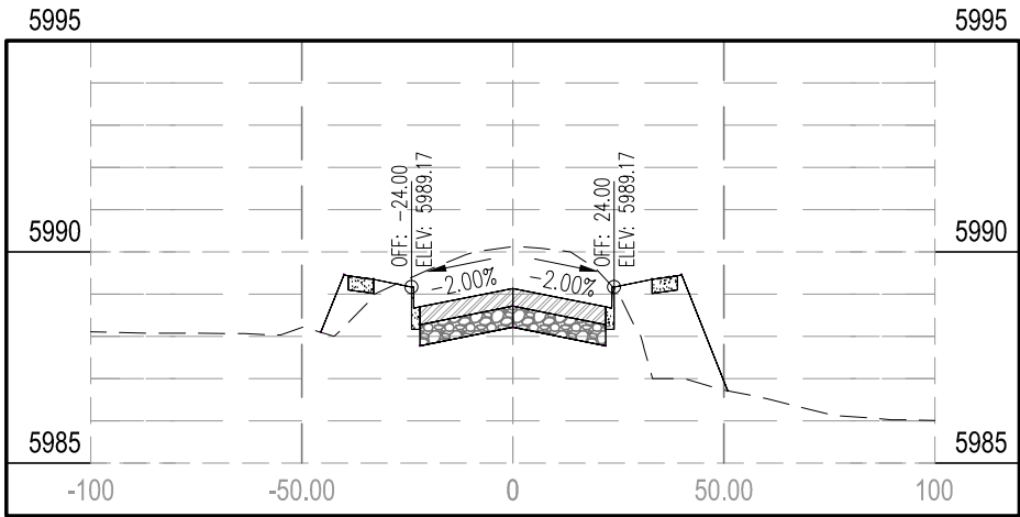
STA 111+00.00
