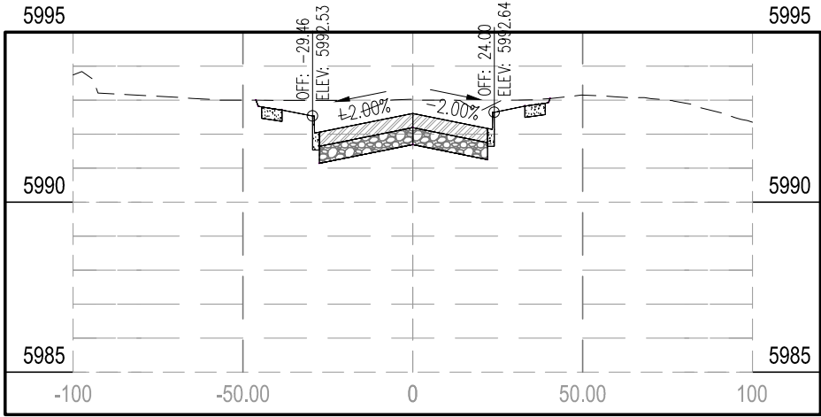
STA 115+00.00
