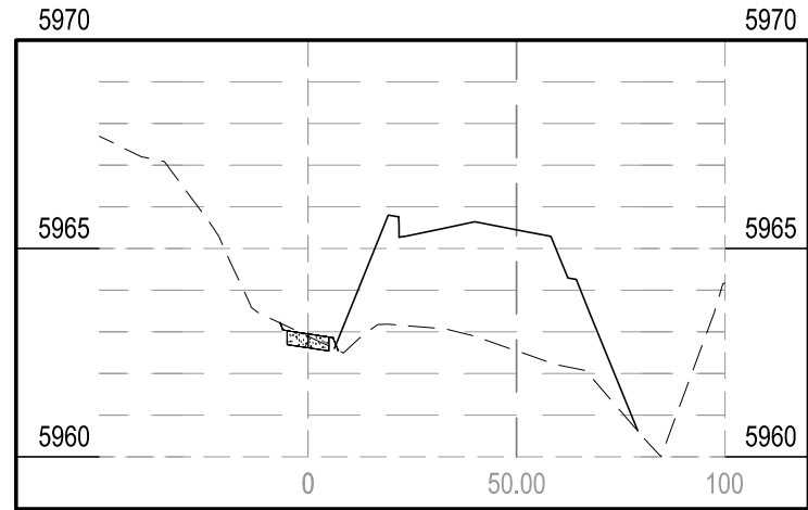
STA 5+50.00
