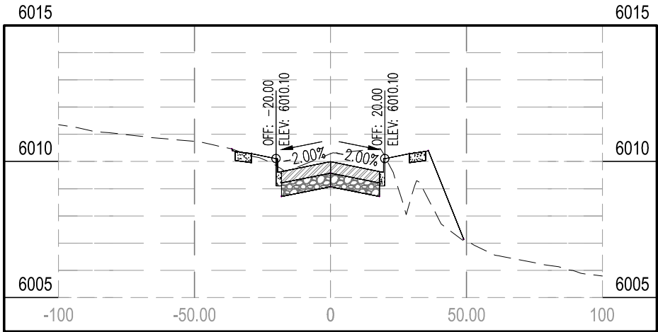
STA 4+51.50
