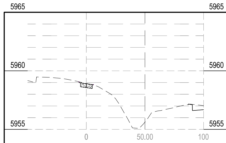
STA 24+50.00
