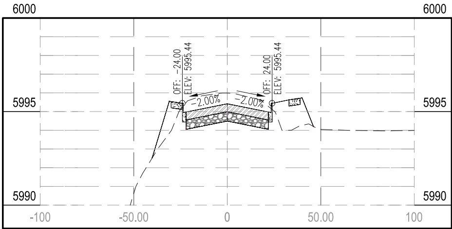
STA 93+00.00
