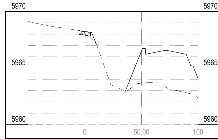
STA 3+50.00
