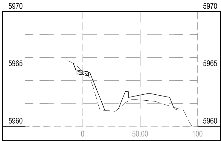
STA 11+00.00
