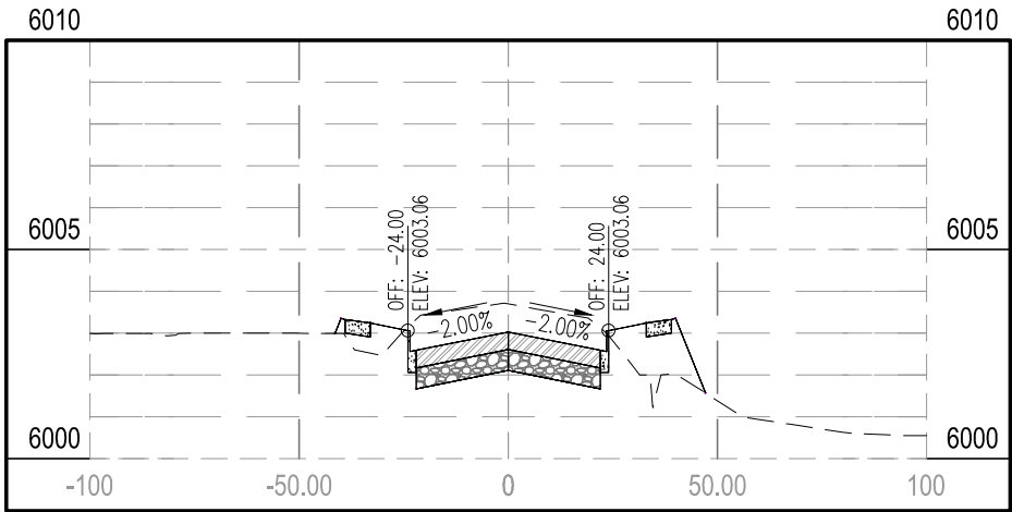
STA 66+00.00
