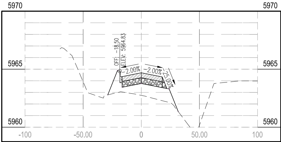
STA 8+00.00
