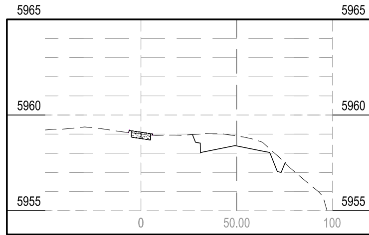
STA 23+50.00
