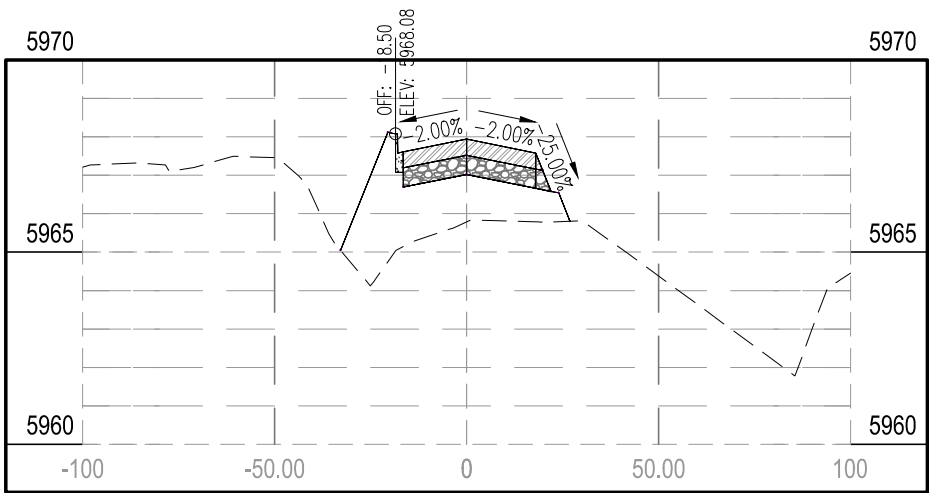
STA 1+50.00
