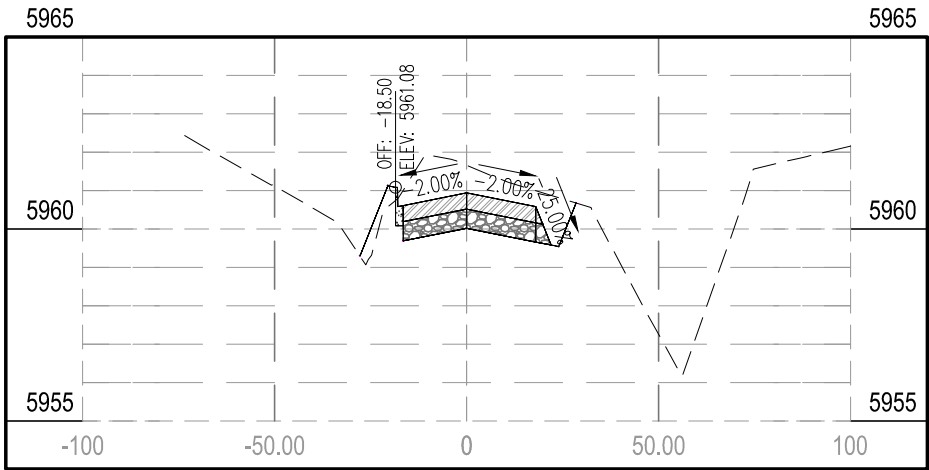
STA 15+50.00
