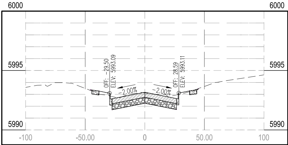
STA 116+00.00
