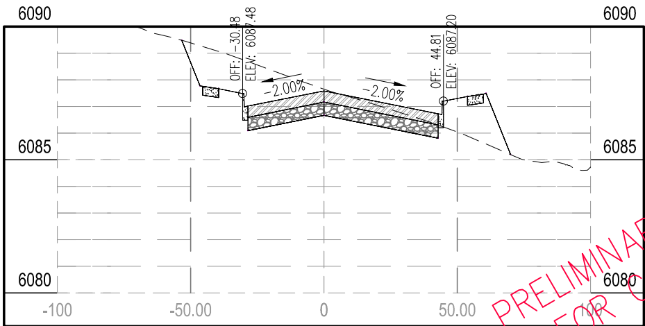
STA 22+00.00
