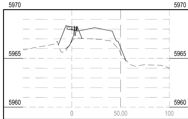
STA 0+68.92
