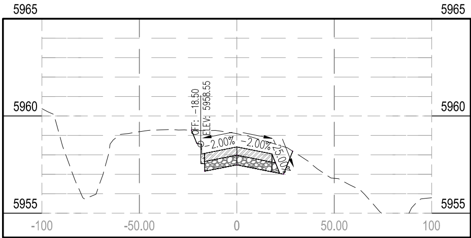
STA 23+50.00
