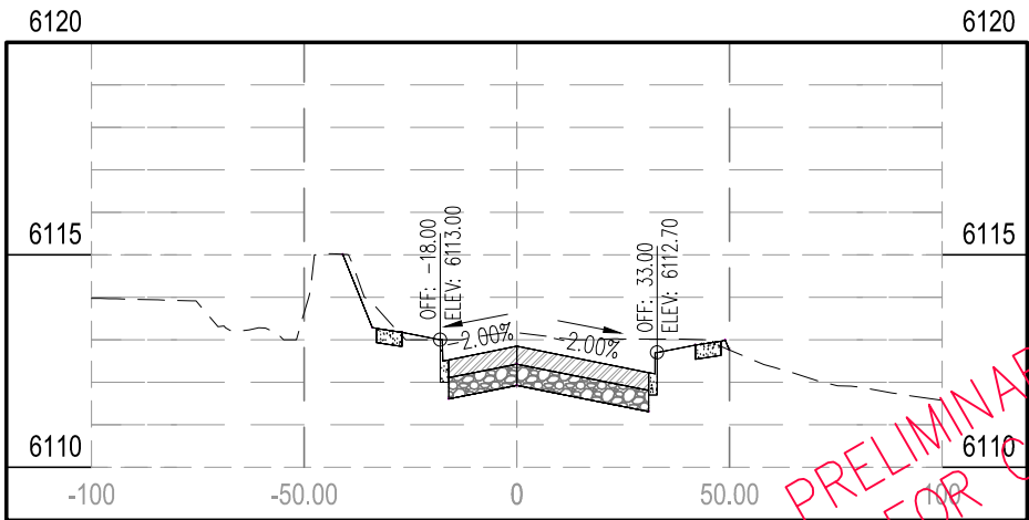
STA 10+00.00
