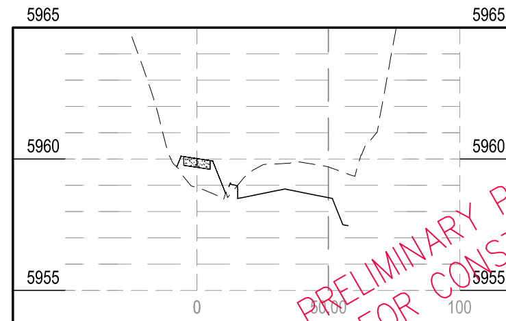
STA 19+12.67
