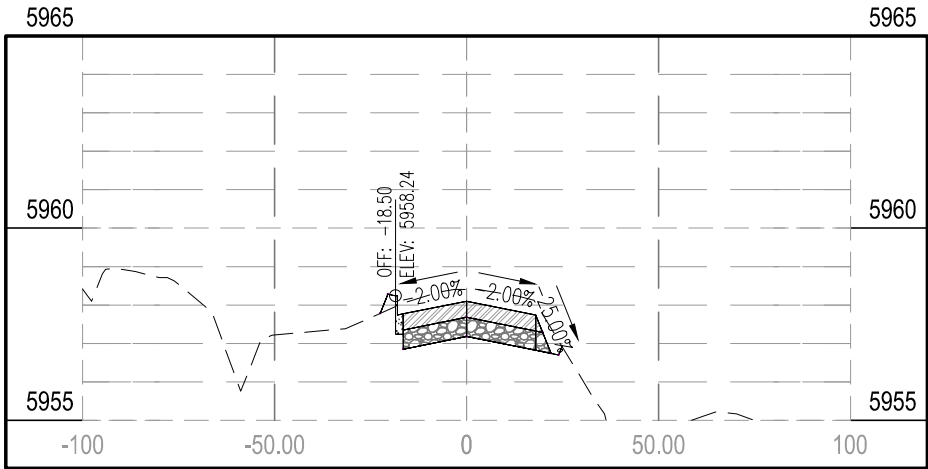
STA 24+50.00
