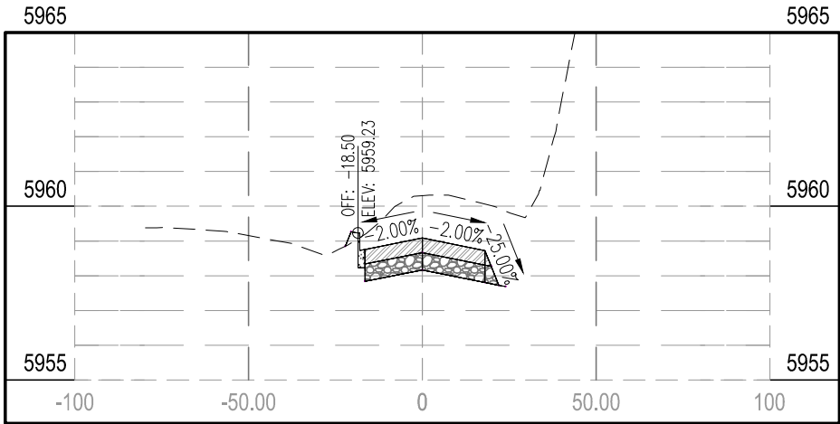
STA 19+21.35
