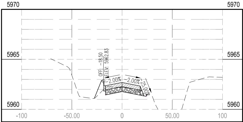
STA 12+00.00
