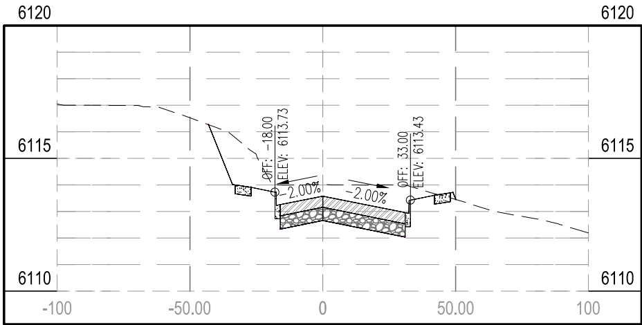
STA 9+00.00
