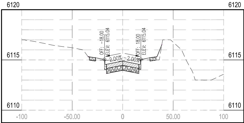
STA 2+00.00
