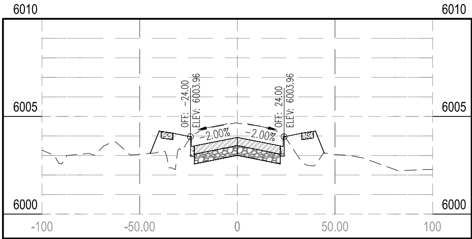
STA 63+00.00
