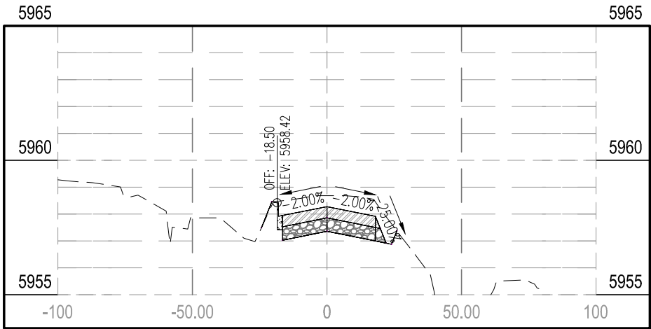
STA 24+25.00
