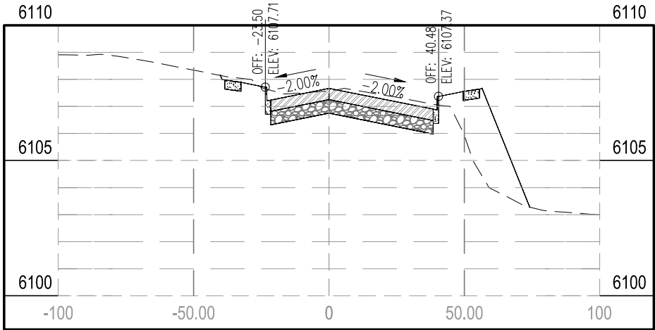
STA 17+00.00
