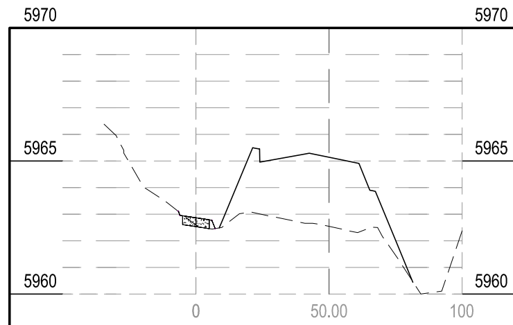
STA 6+02.55
