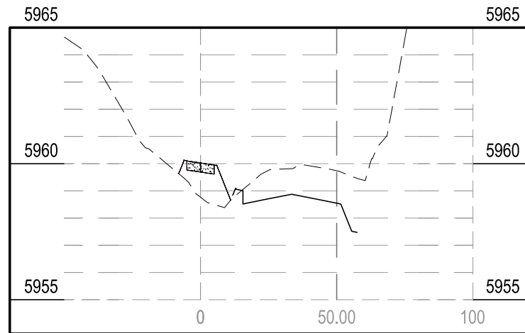
STA 19+05.84
