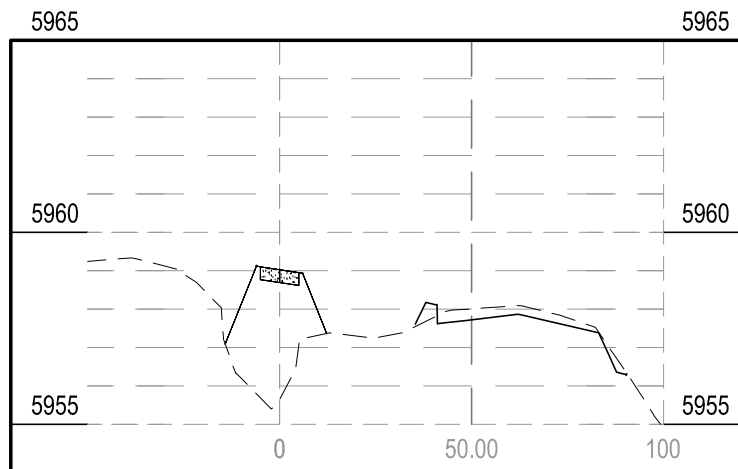
STA 23+86.49
