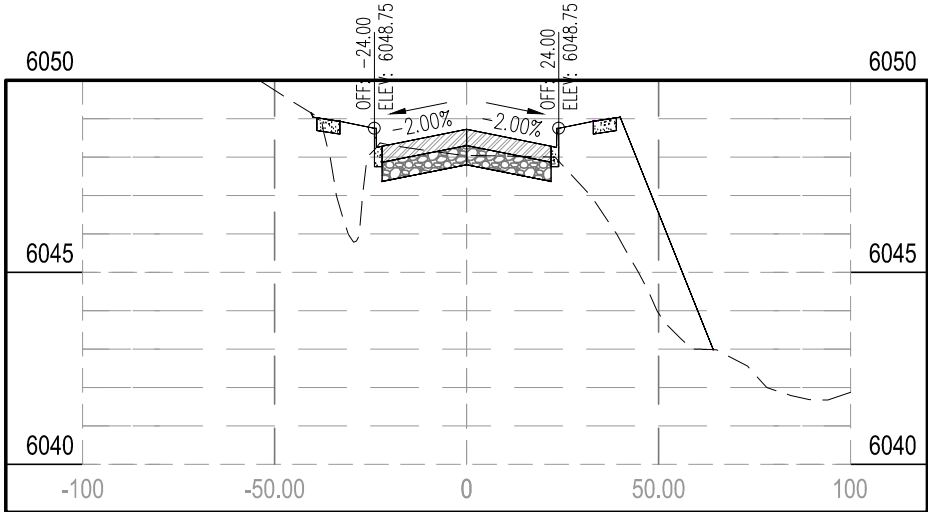
STA 37+00.00
