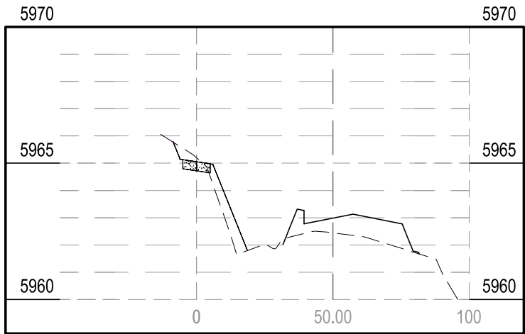
STA 10+50.00
