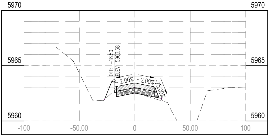
STA 10+50.00
