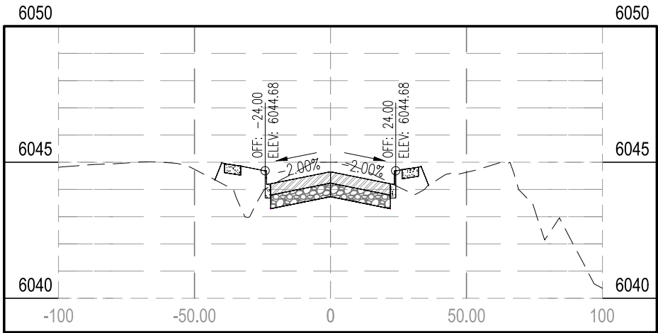
STA 42+00.00
