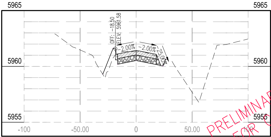
STA 14+50.00
