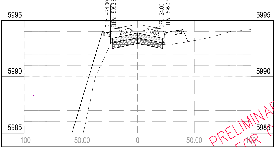
STA 100+00.00
