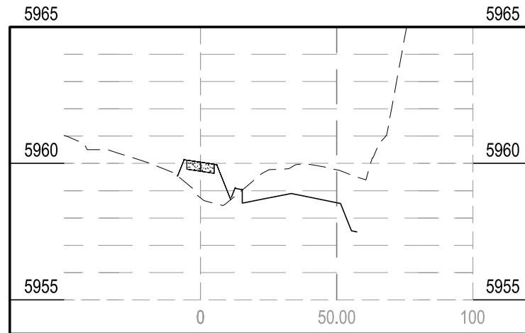
STA 19+00.00
