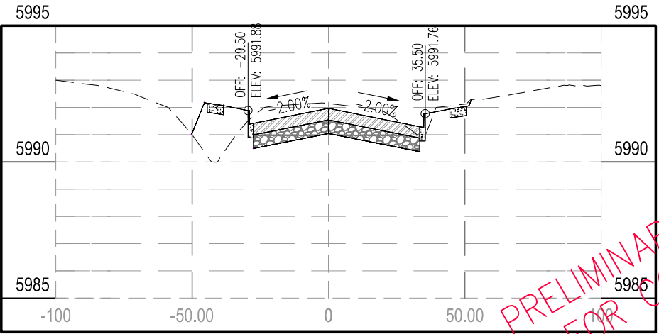
STA 118+00.00
