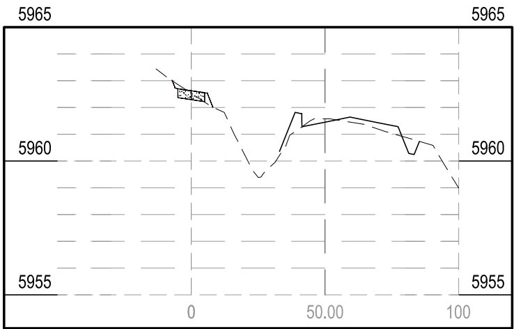
STA 13+50.00
