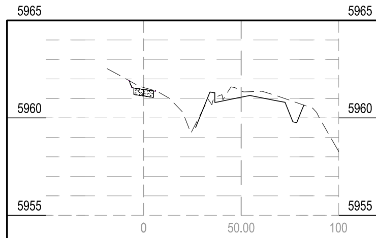
STA 14+50.00
