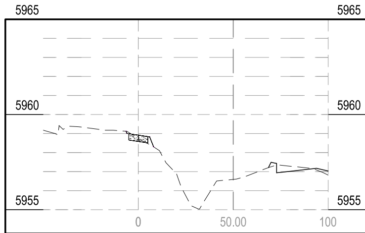
STA 24+39.20
