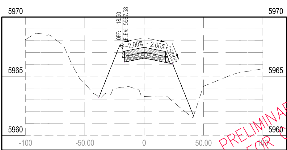
STA 2+50.00
