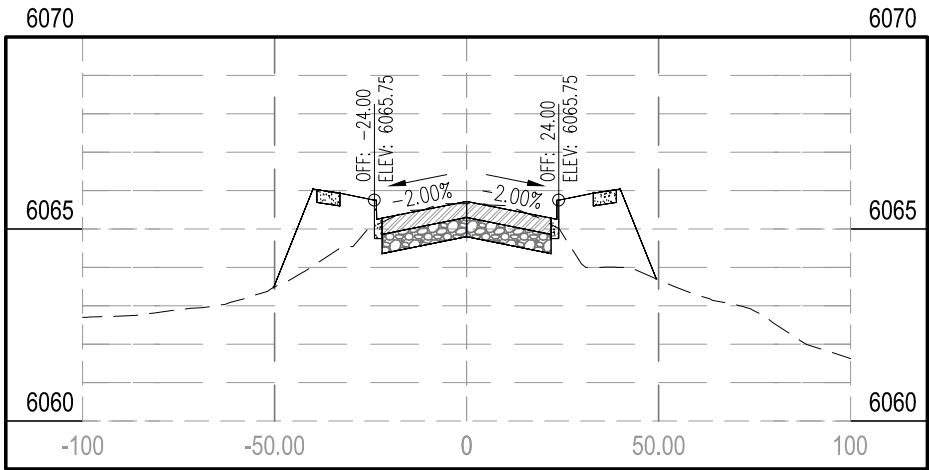
STA 30+00.00
