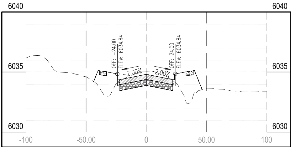
STA 49+00.00
