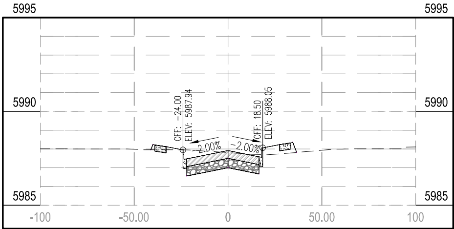
STA 125+00.00
