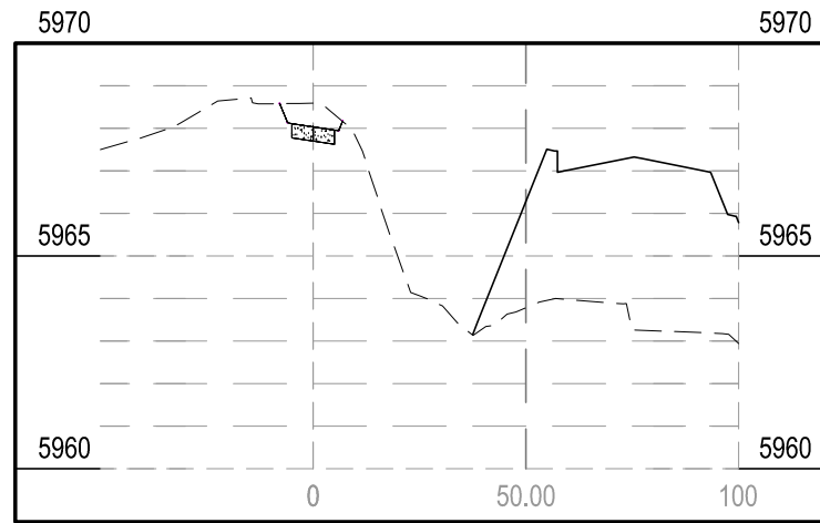
STA 2+00.00
