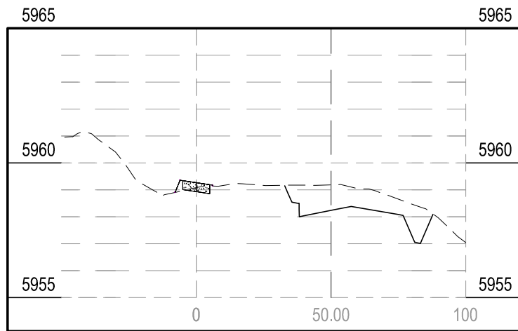
STA 22+72.32
