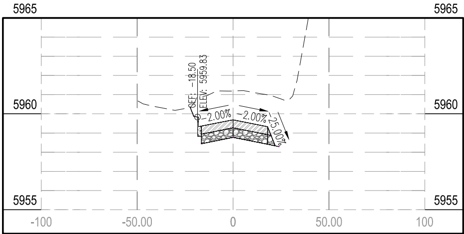
STA 18+00.00
