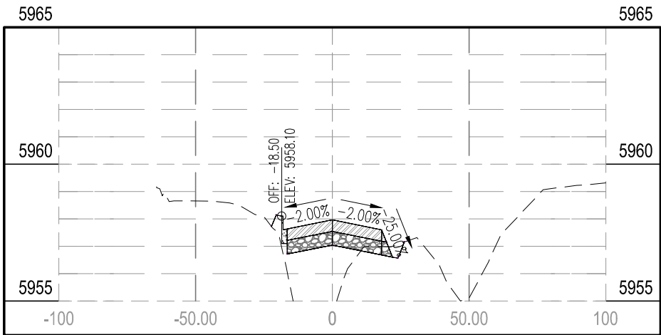
STA 22+50.00
