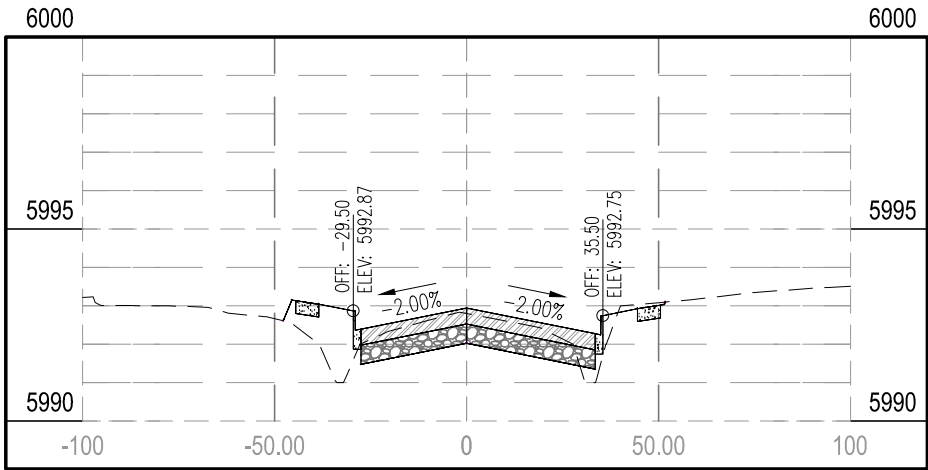
STA 117+00.00
