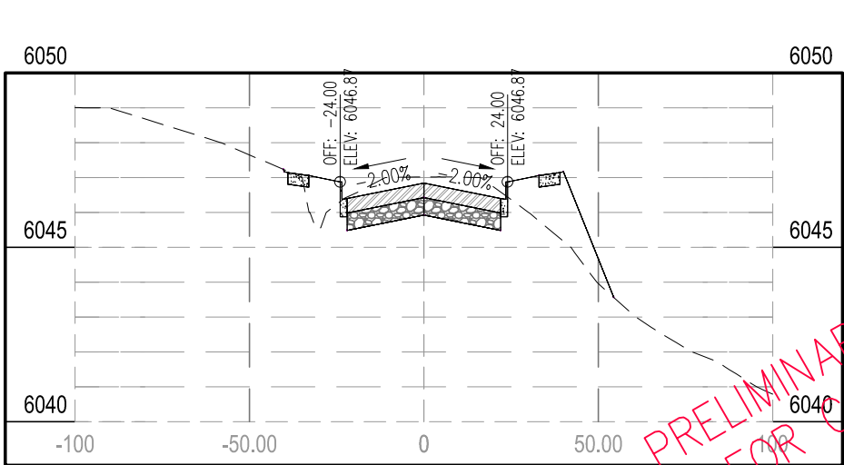
STA 40+00.00
