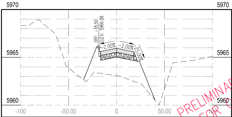
STA 5+50.00
