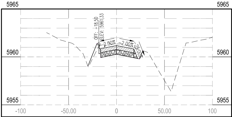
STA 15+00.00
