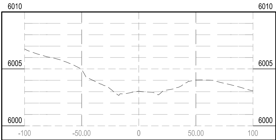
STA 0+00.00
