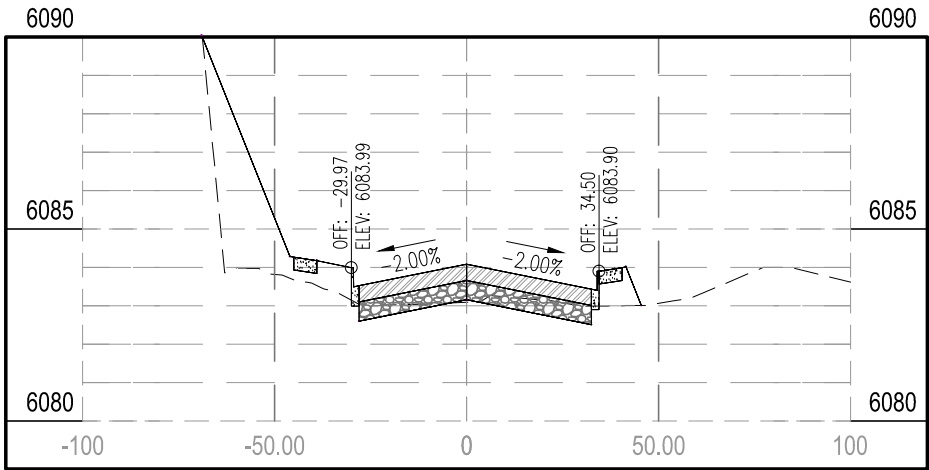
STA 24+00.00
