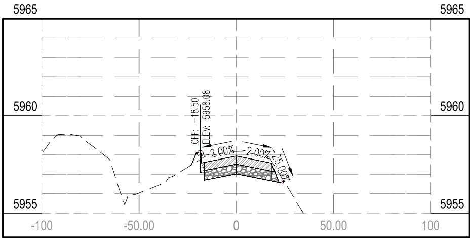
STA 24+67.10
