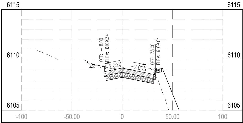
STA 15+00.00
