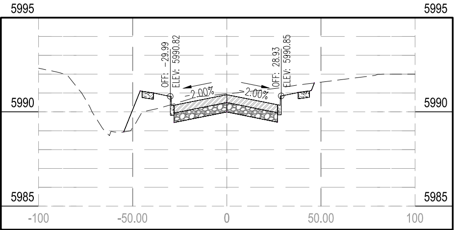
STA 119+00.00
