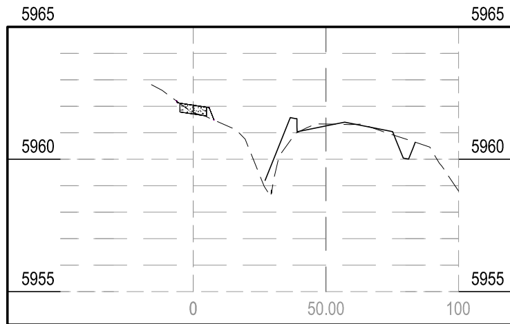
STA 14+00.00
