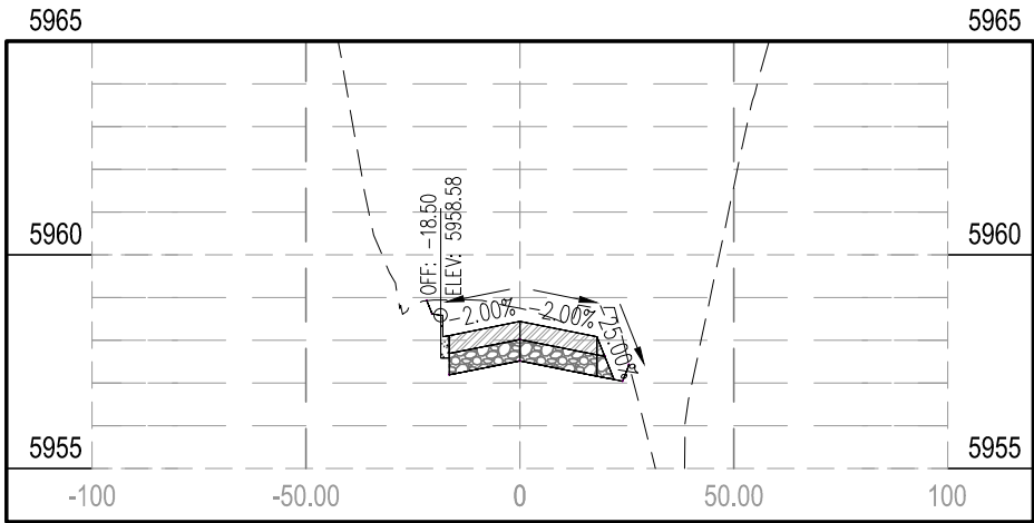
STA 20+50.00
