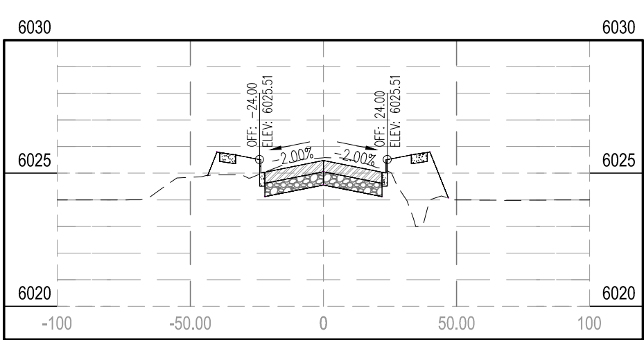
STA 53+00.00
