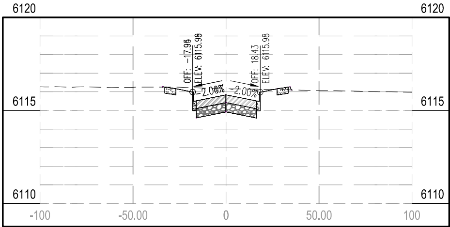
STA 3+00.00
