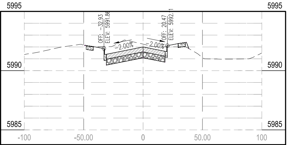
STA 120+00.00
