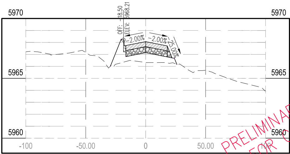
STA 1+25.00
