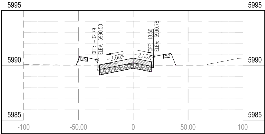
STA 122+00.00
