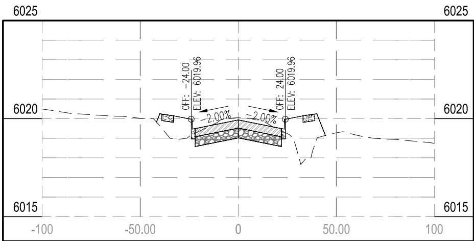
STA 55+00.00
