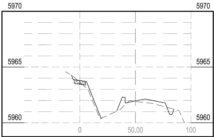
STA 12+50.00
