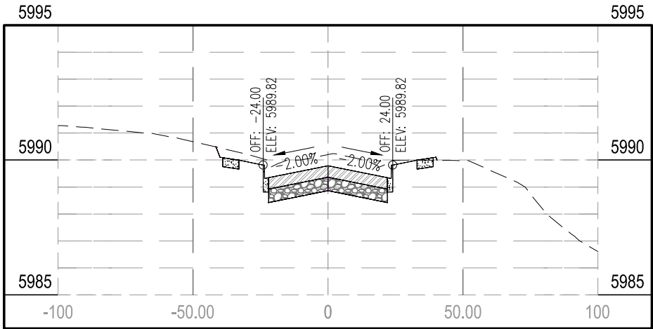
STA 113+00.00
