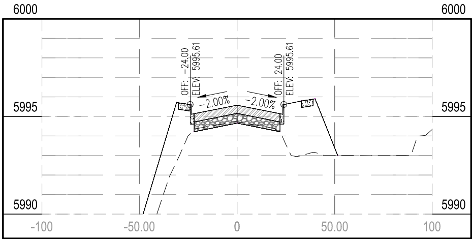
STA 96+00.00
