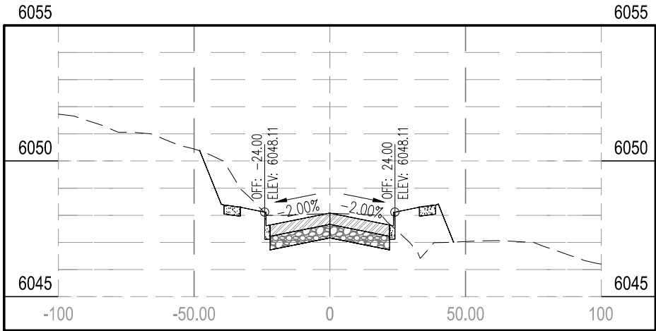
STA 38+00.00
