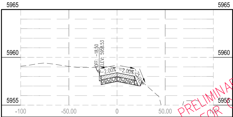
STA 23+98.76
