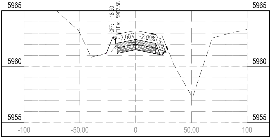
STA 12+50.00
