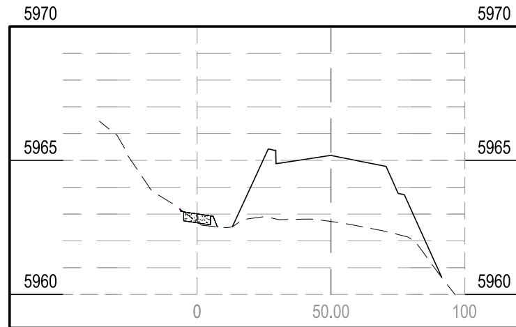
STA 6+09.75
