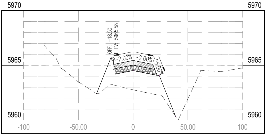
STA 6+50.00
