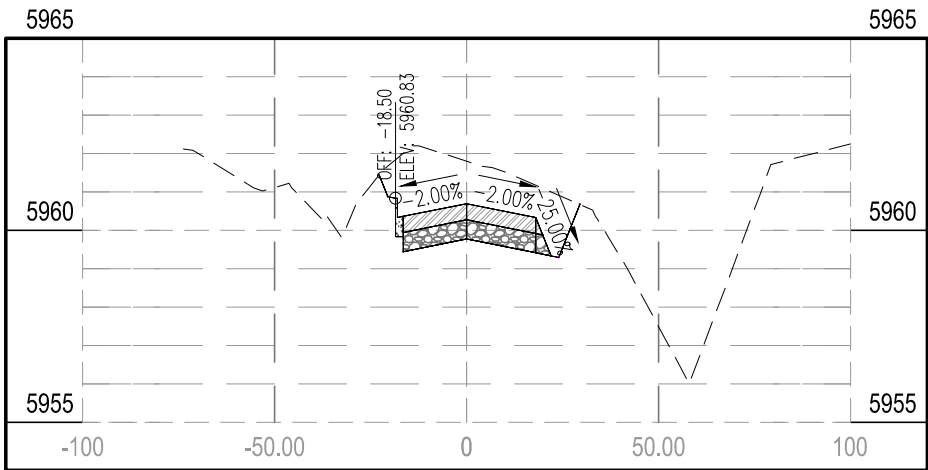
STA 16+00.00
