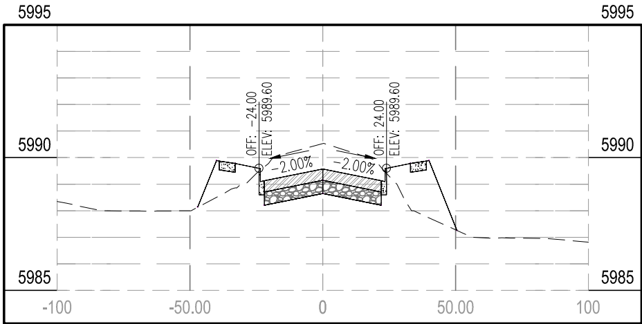
STA 110+00.00
