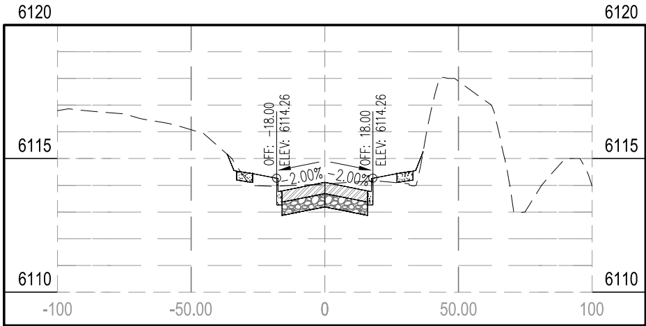
STA 1+50.00
