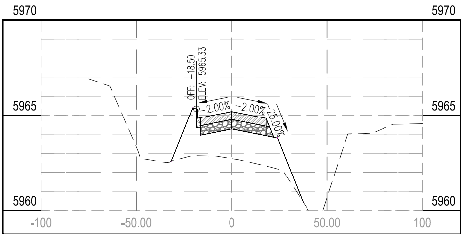
STA 7+00.00
