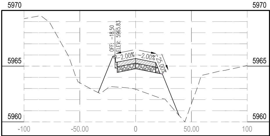
STA 6+00.00
