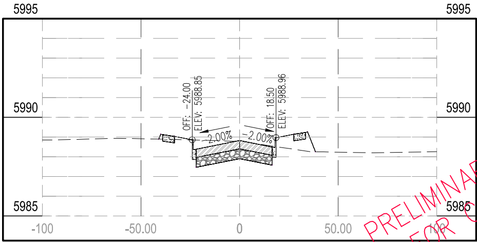
STA 124+00.00
