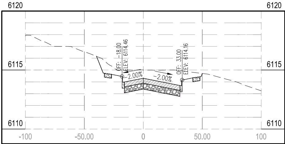
STA 8+00.00
