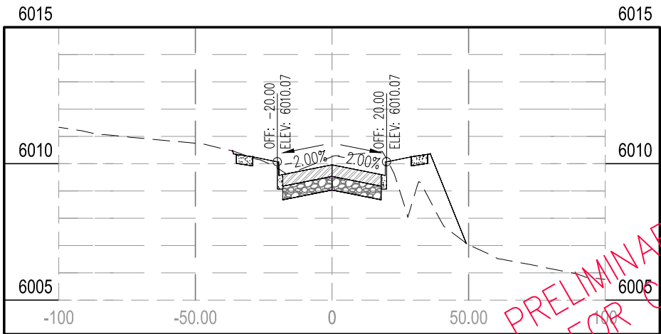
STA 4+50.00
