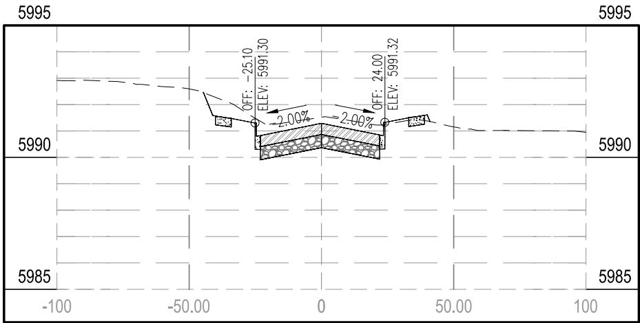
STA 114+00.00
