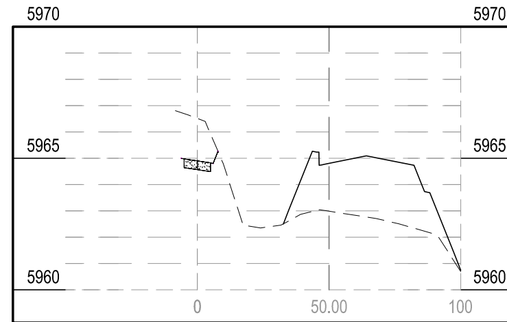
STA 6+60.06
