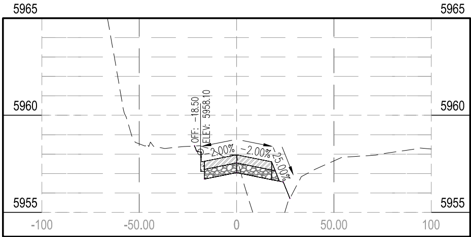
STA 21+50.00
