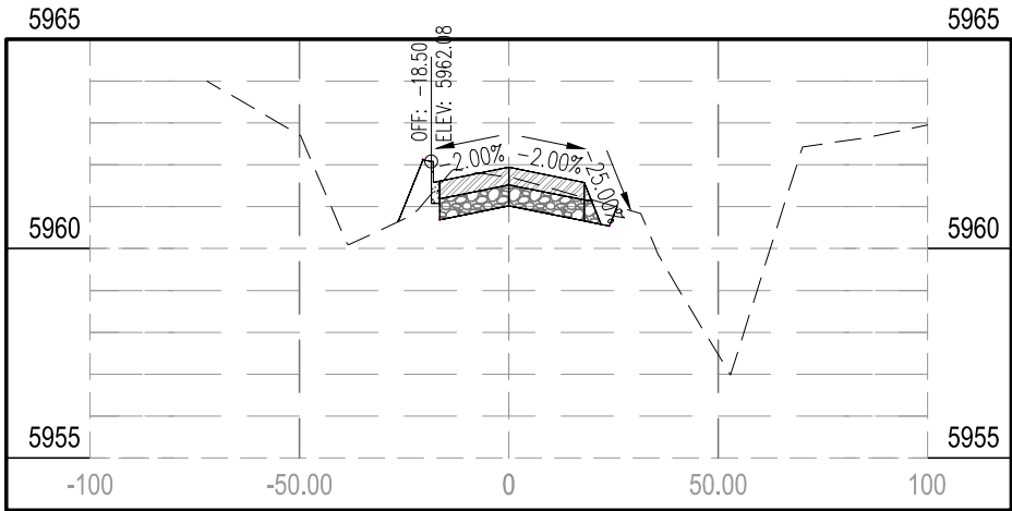
STA 13+50.00
