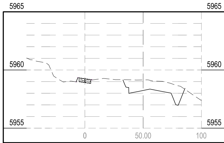
STA 22+79.40
