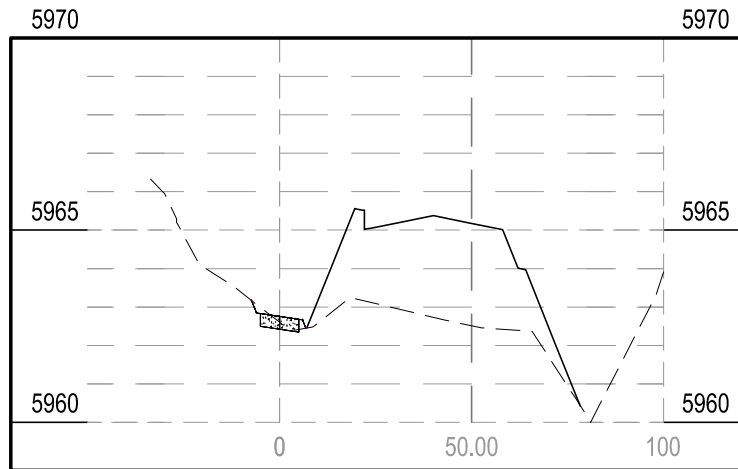
STA 5+95.35
