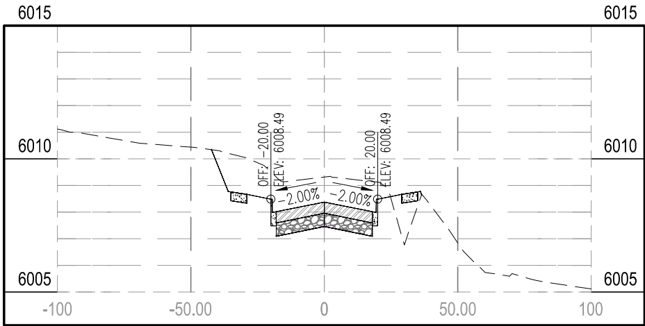
STA 4+00.00
