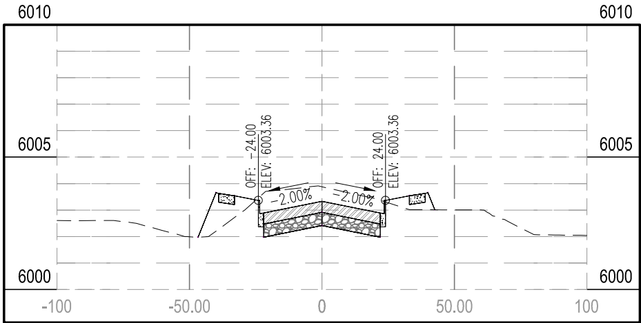
STA 65+00.00
