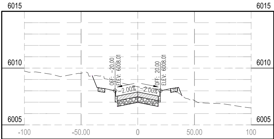
STA 3+00.00
