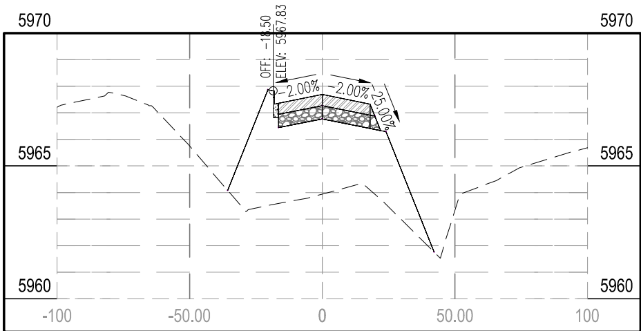
STA 2+00.00
