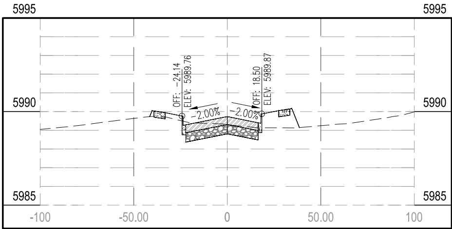
STA 123+00.00
