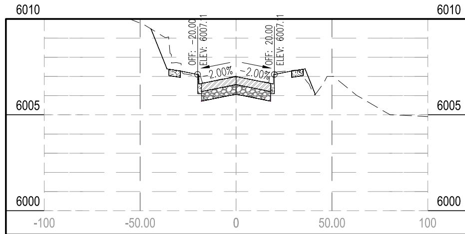
STA 2+00.00
