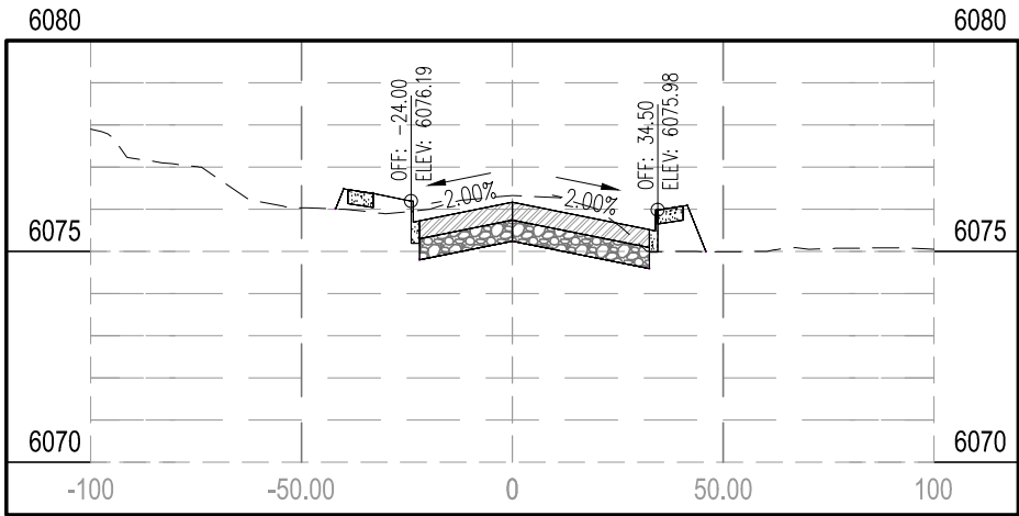
STA 27+00.00
