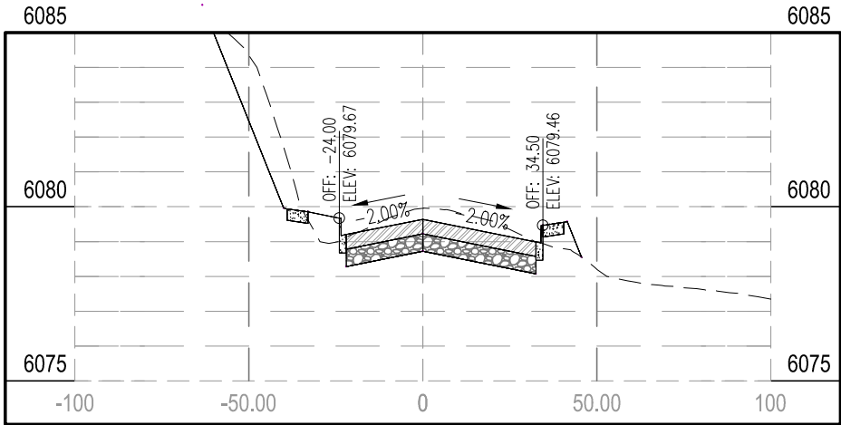
STA 26+00.00
