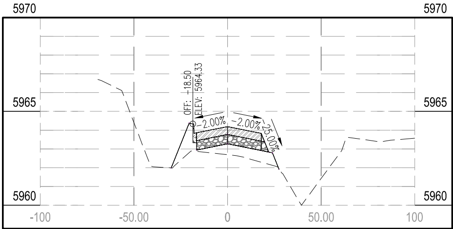
STA 9+00.00
