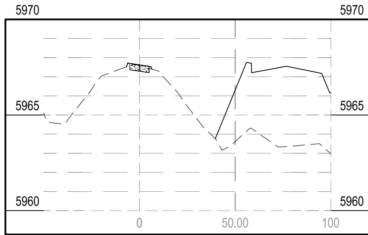
STA 1+38.09
