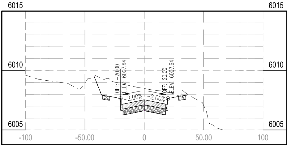
STA 3+50.00
