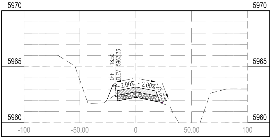
STA 11+00.00
