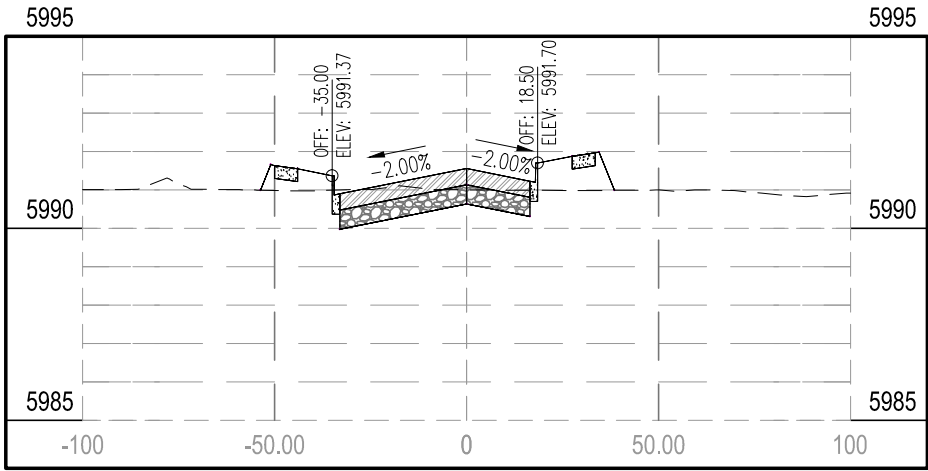
STA 121+00.00
