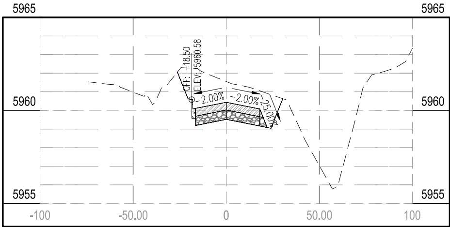
STA 16+50.00
