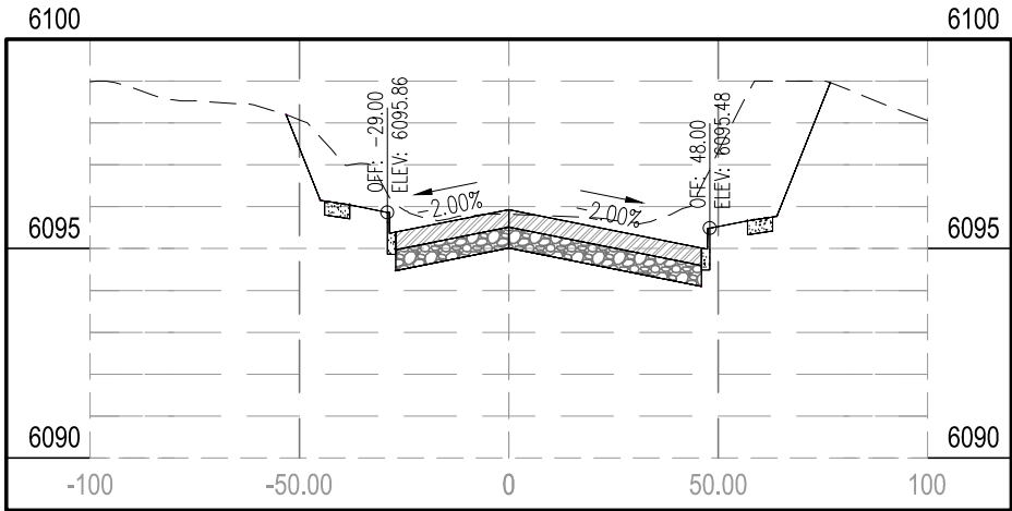
STA 20+00.00
