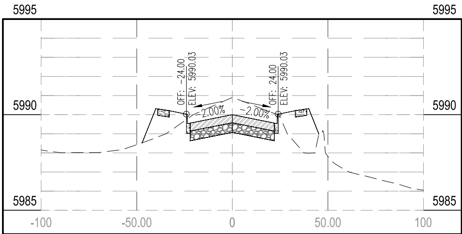
STA 109+00.00
