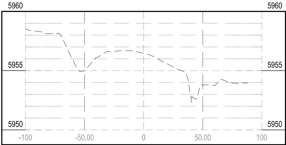
STA 26+00.00
