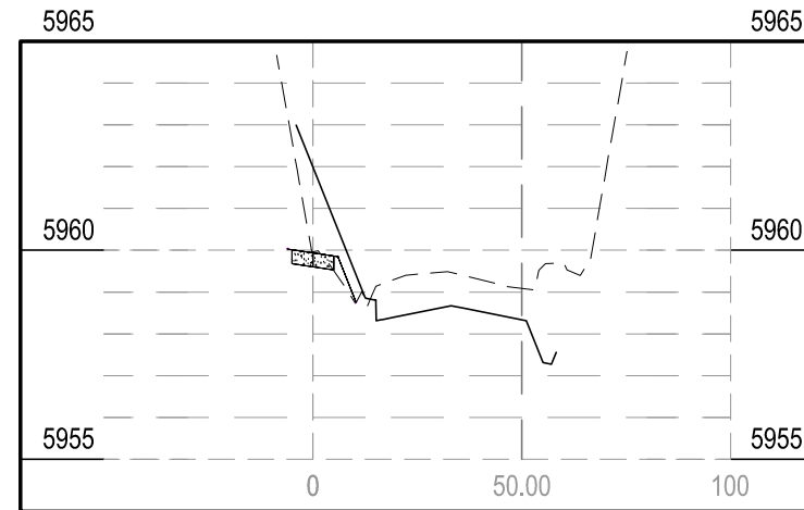
STA 19+50.00
