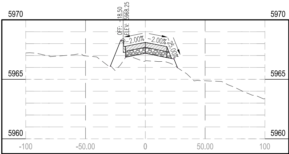
STA 1+16.50
