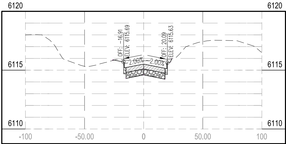
STA 3+50.00
