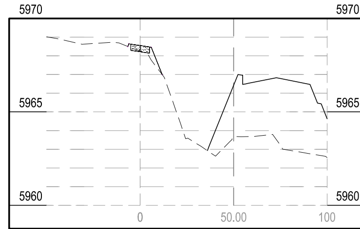
STA 3+00.00
