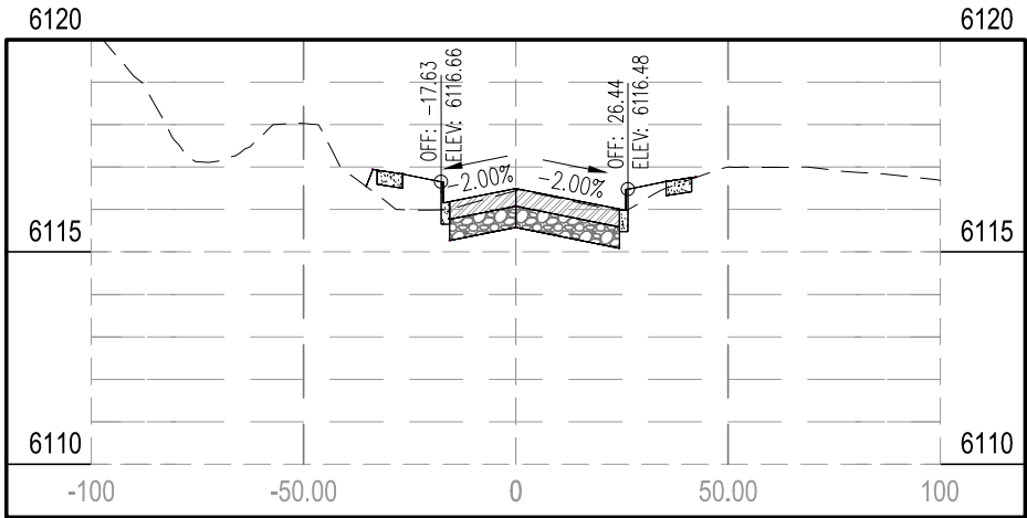
STA 5+00.00
