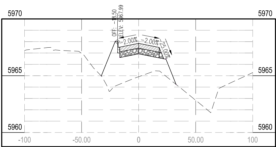
STA 1+68.51
