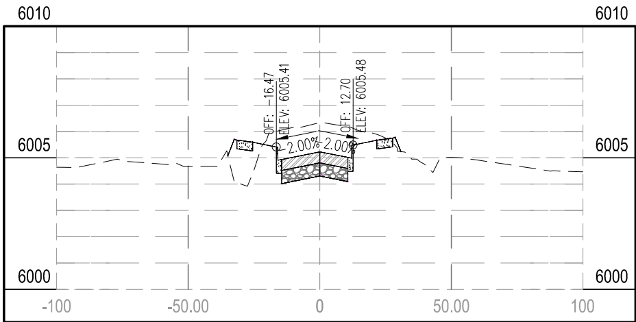
STA 61+00.00
