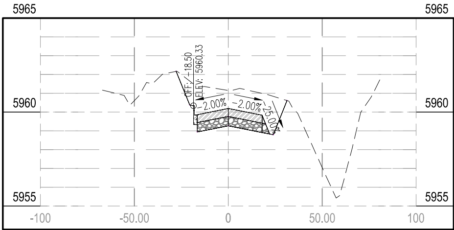
STA 17+00.00
