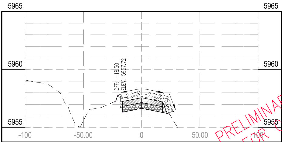
STA 25+00.00
