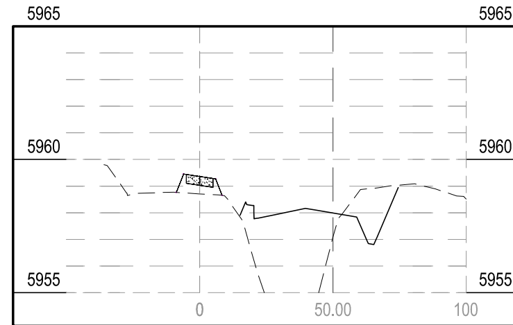
STA 22+26.08
