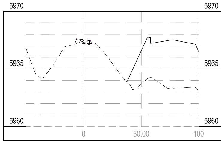
STA 1+25.00
