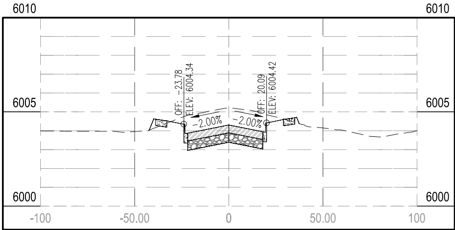
STA 62+00.00
