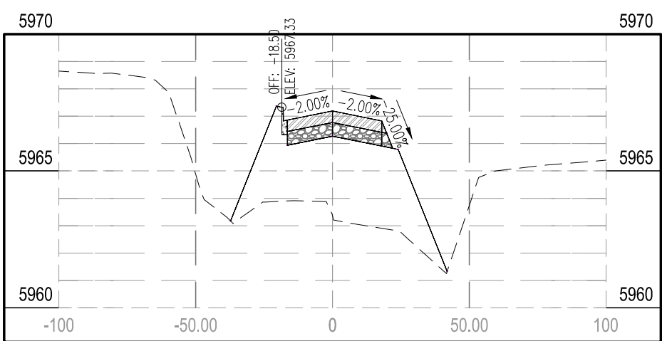
STA 3+00.00
