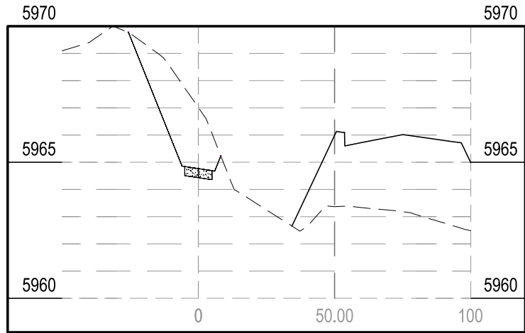
STA 5+02.00
