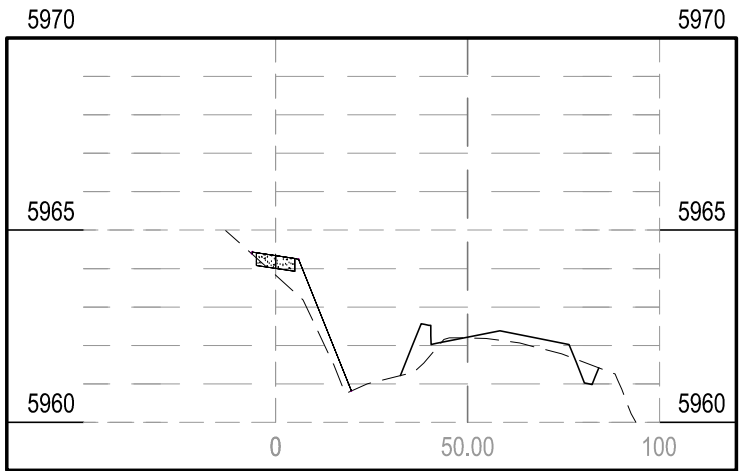
STA 12+00.00
