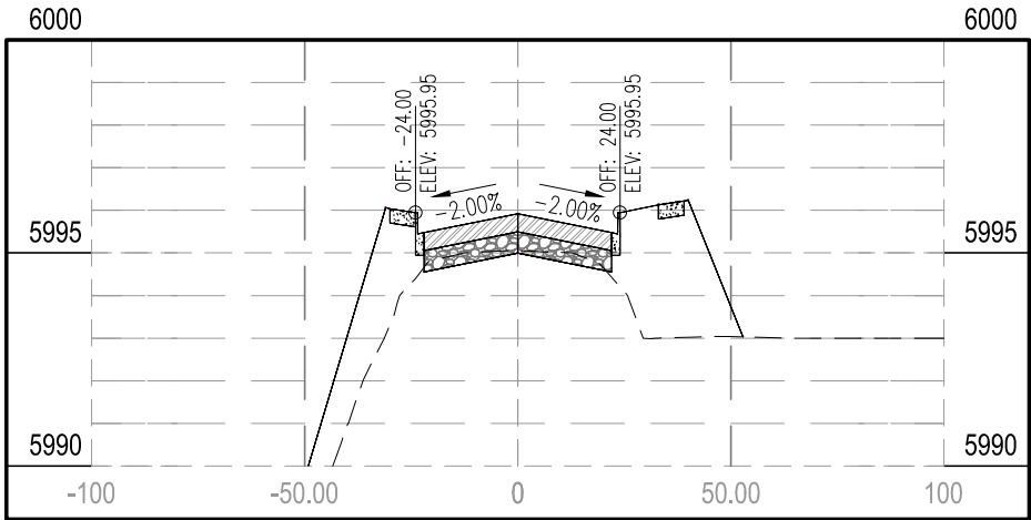
STA 95+00.00
