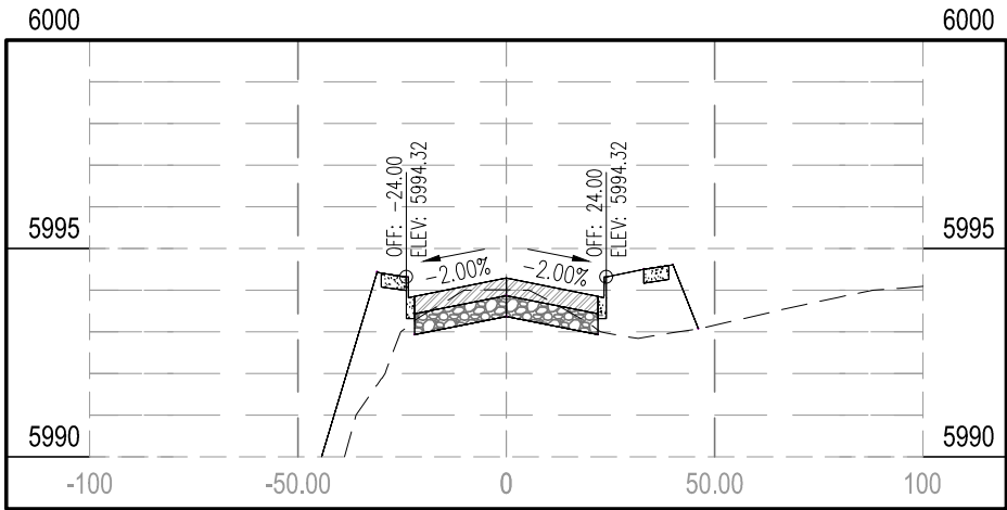
STA 99+00.00
