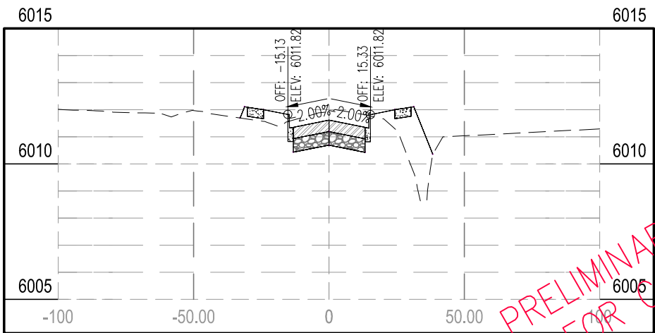
STA 58+00.00
