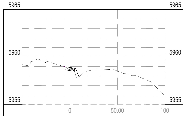
STA 24+75.00
