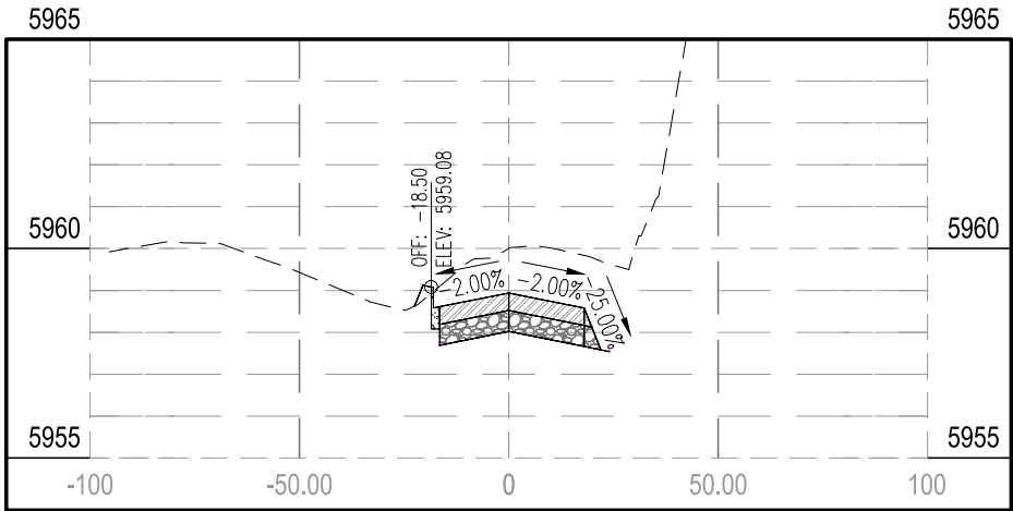
STA 19+50.04
