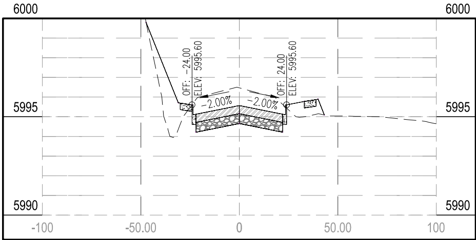
STA 92+00.00
