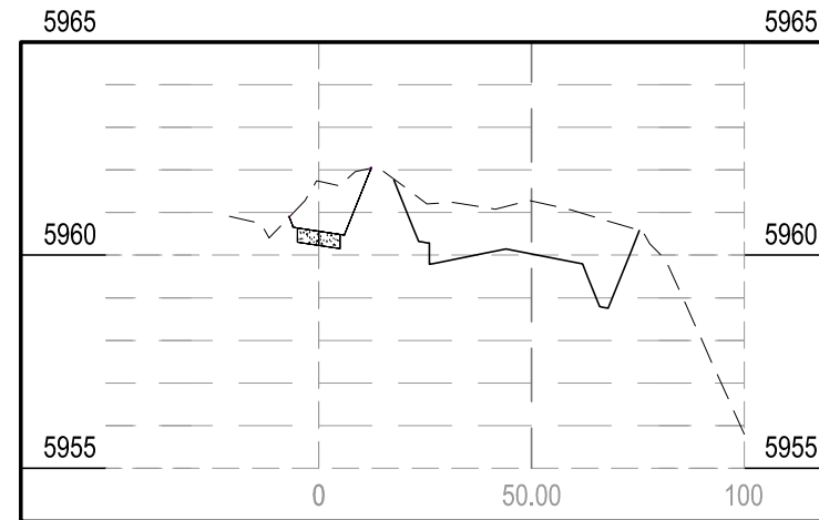
STA 16+50.00
