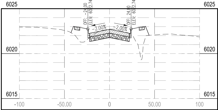
STA 54+00.00
