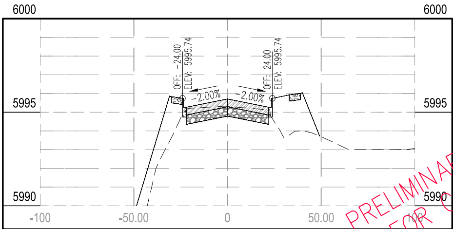
STA 94+00.00
