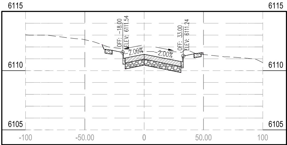
STA 12+00.00
