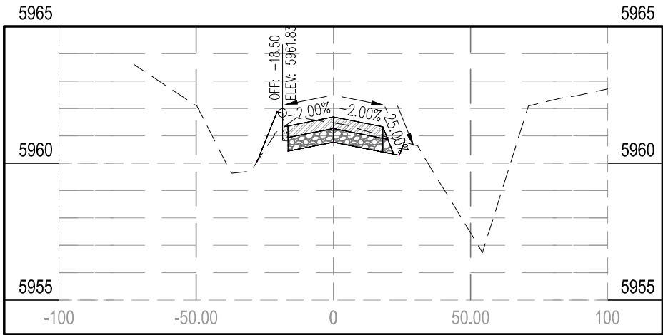
STA 14+00.00
