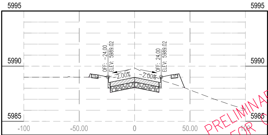
STA 112+00.00
